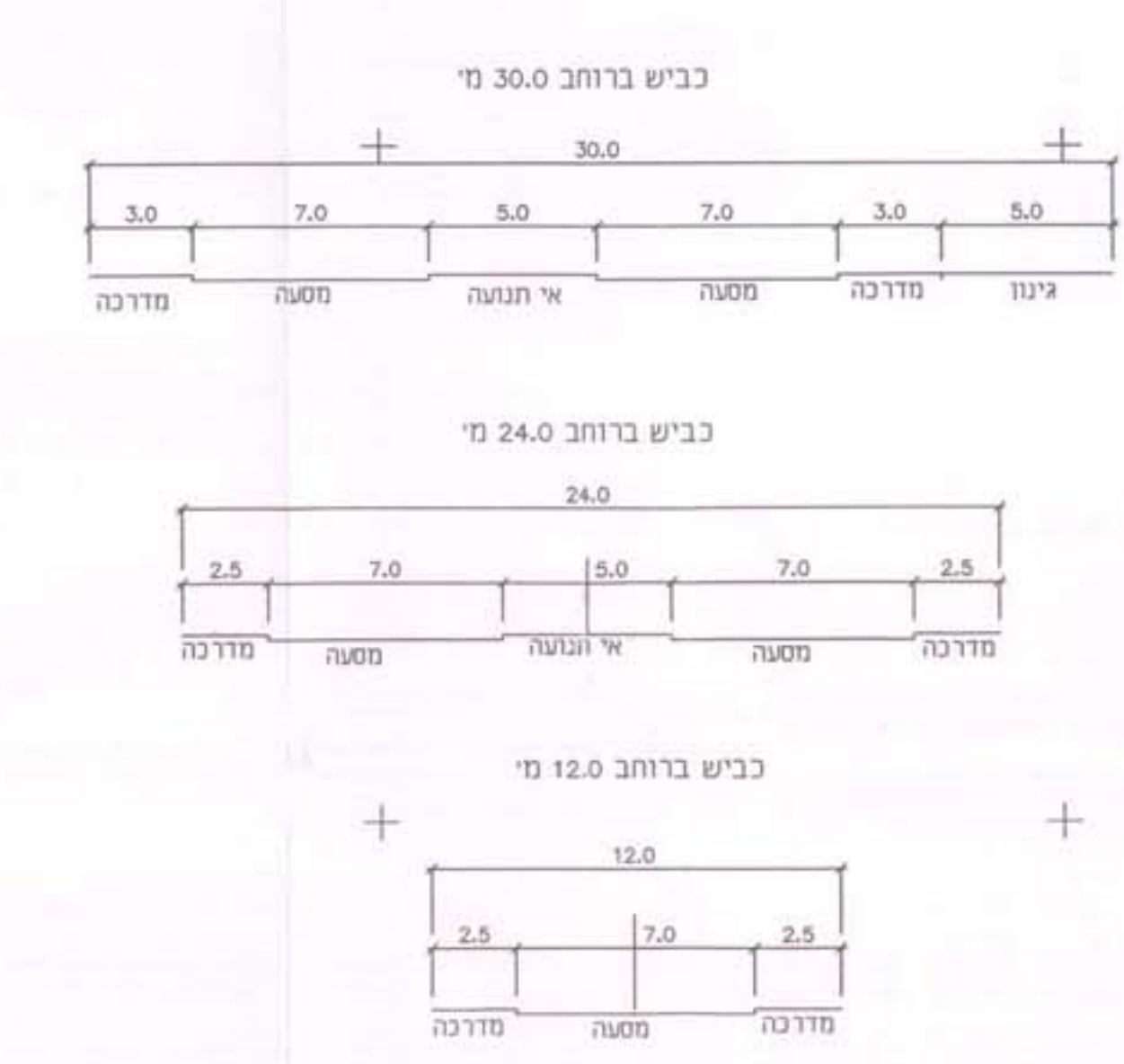
חתכים טיפוסיים לשכונת המגורים
