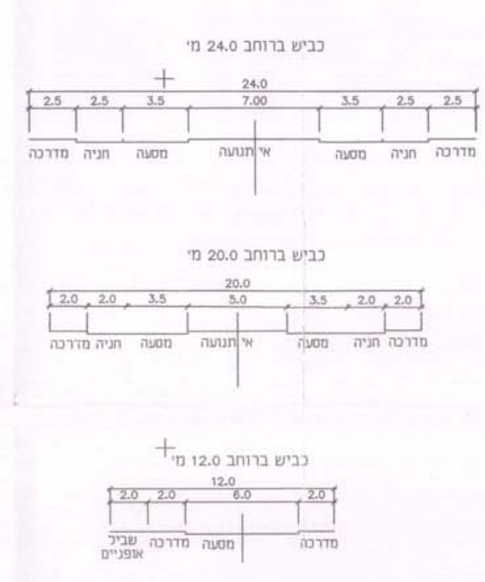
חתכים טיפוסיים למרכז המאבק במדבור
