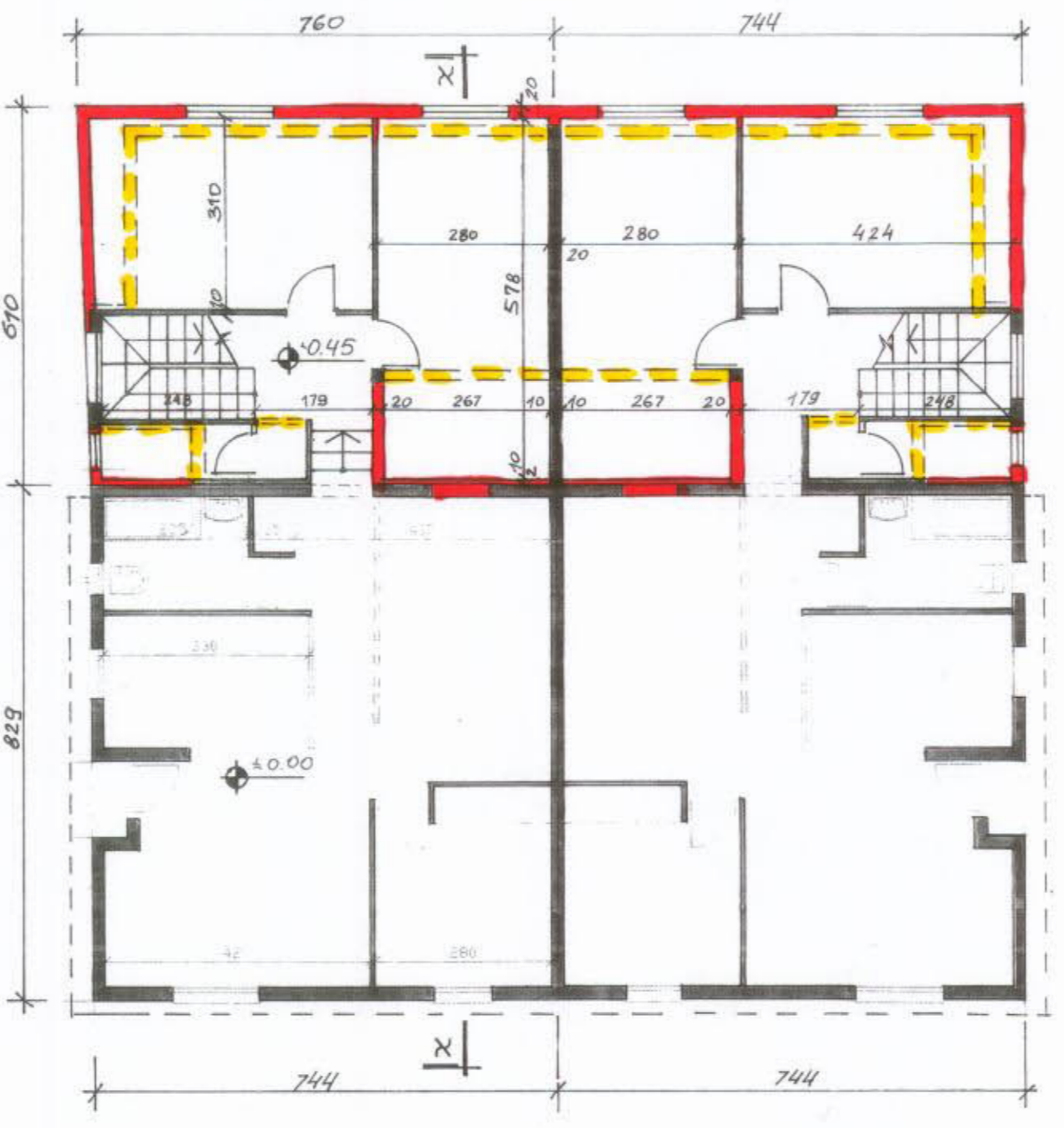
תכנית קומת קרקע קנ"מ 1:100
