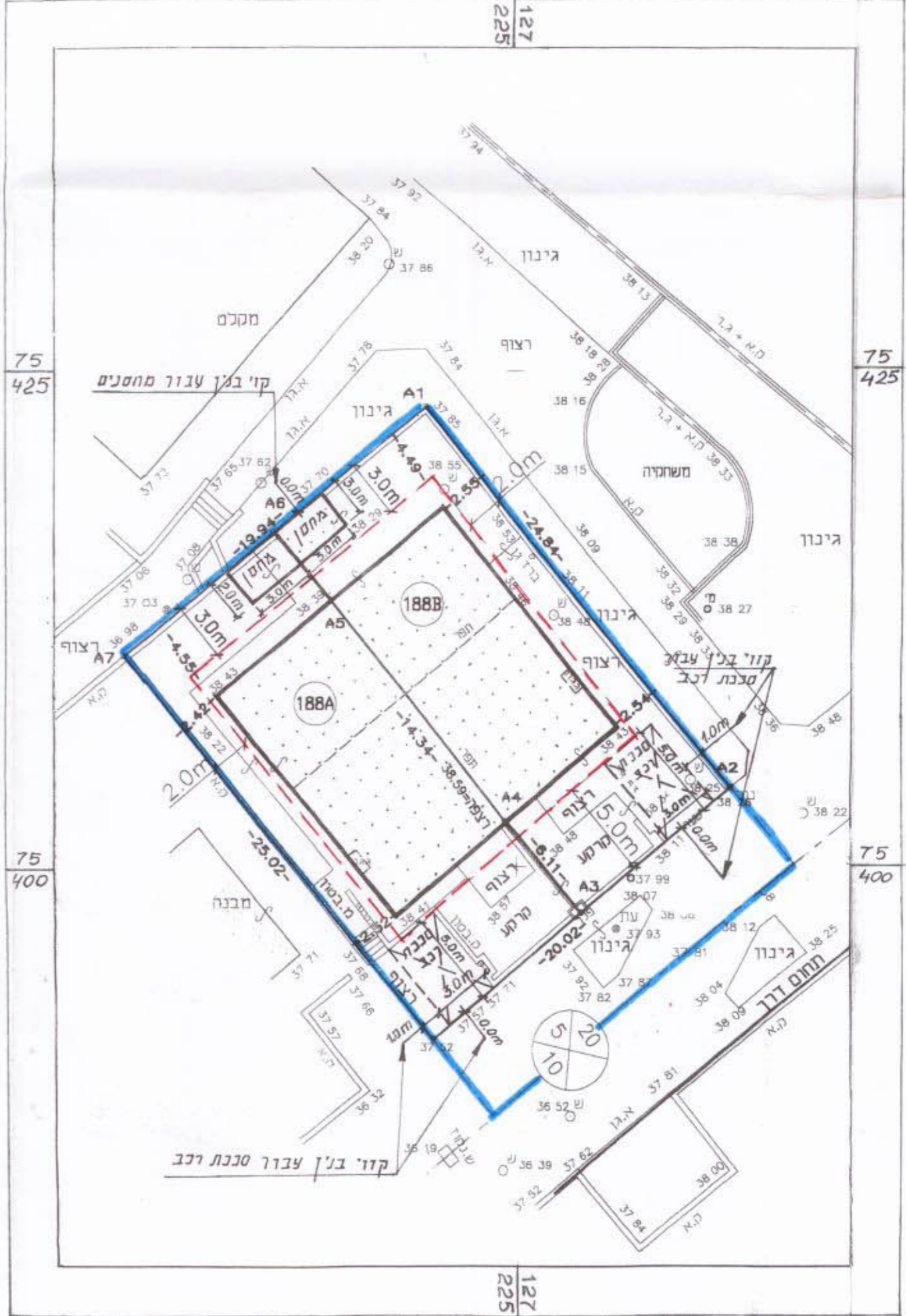
תכנית העמדה קנ"מ 1:250
