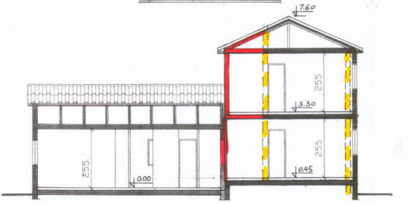
תחר א-א קנ"מ 1:100
