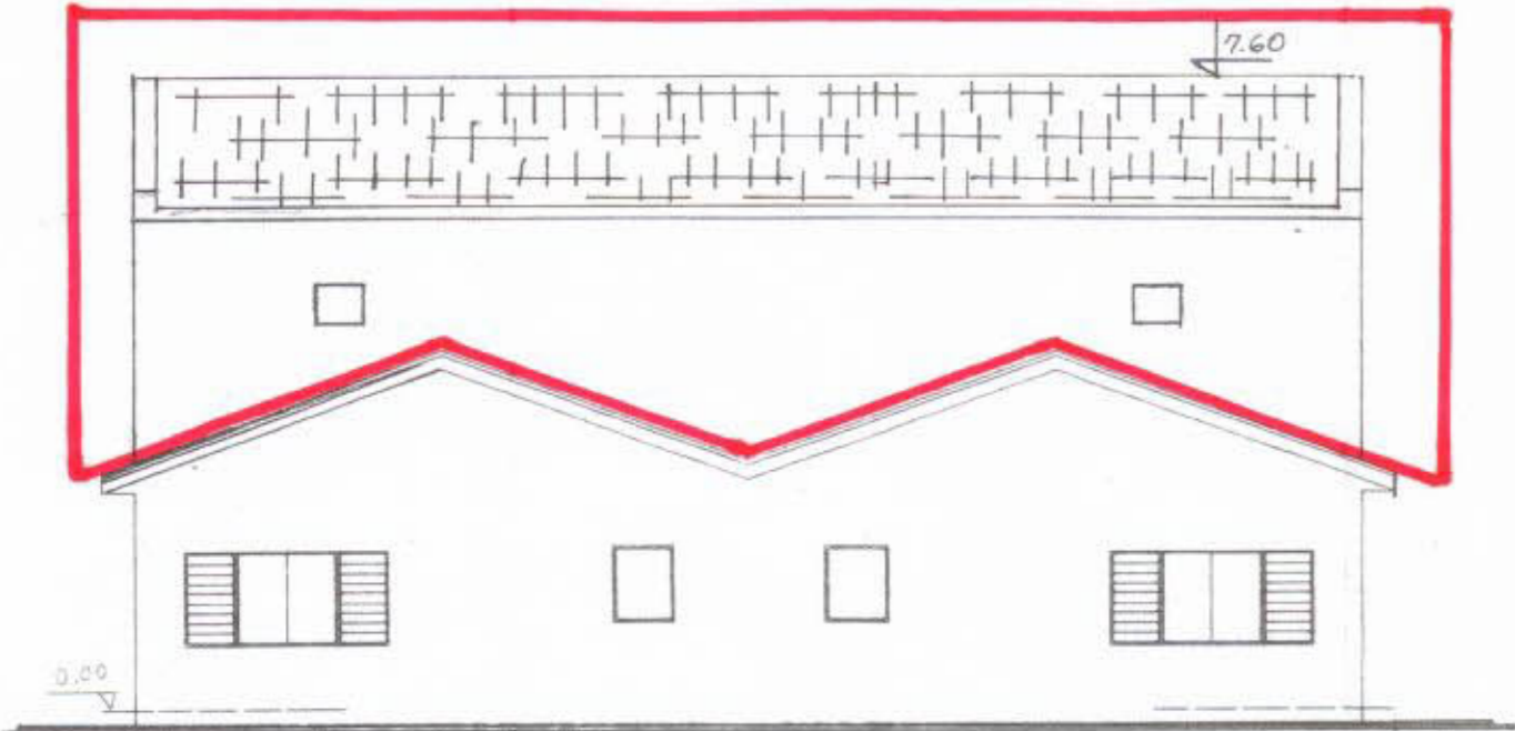
חזית קדמית קנ"מ 1:100
