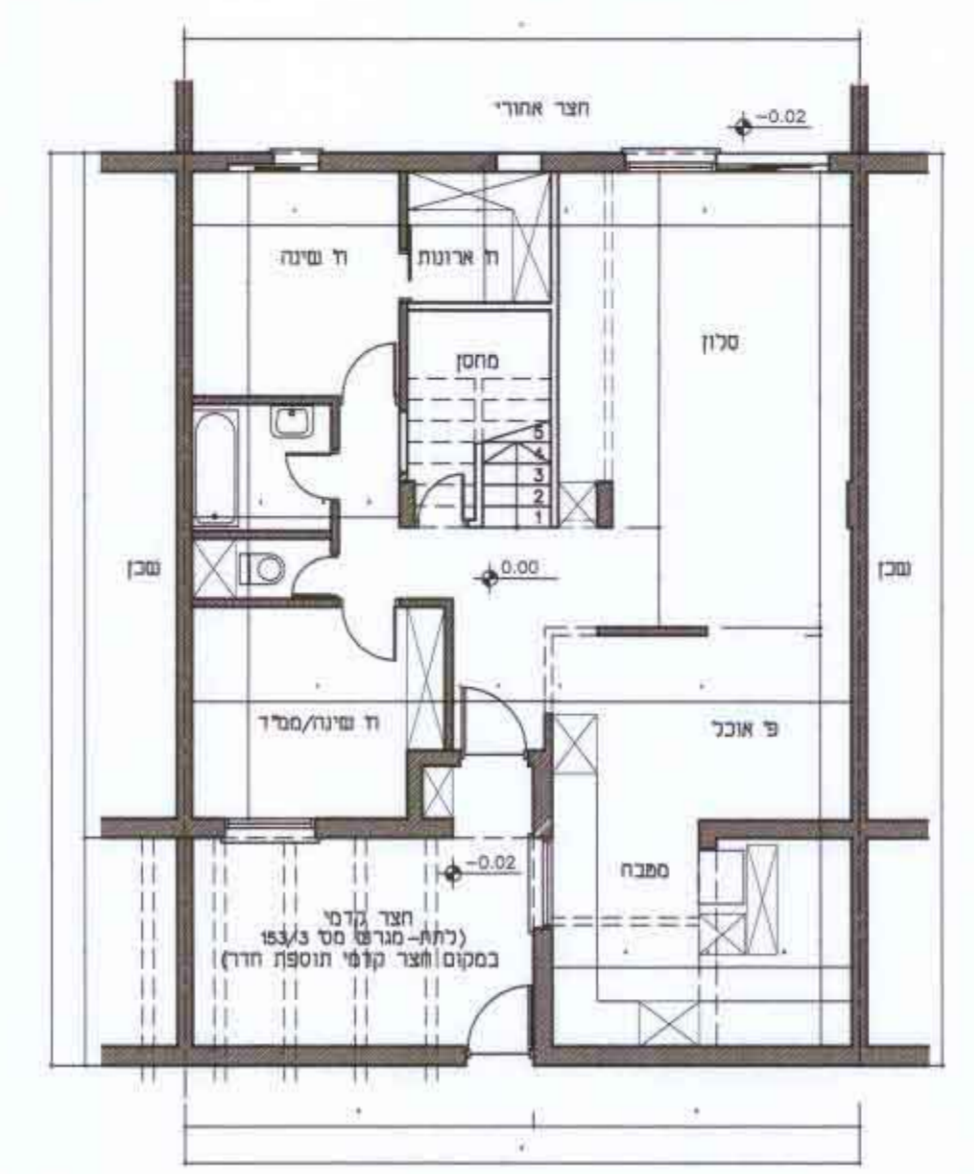
תכנית קומת קרקע קני"מ 1:100
