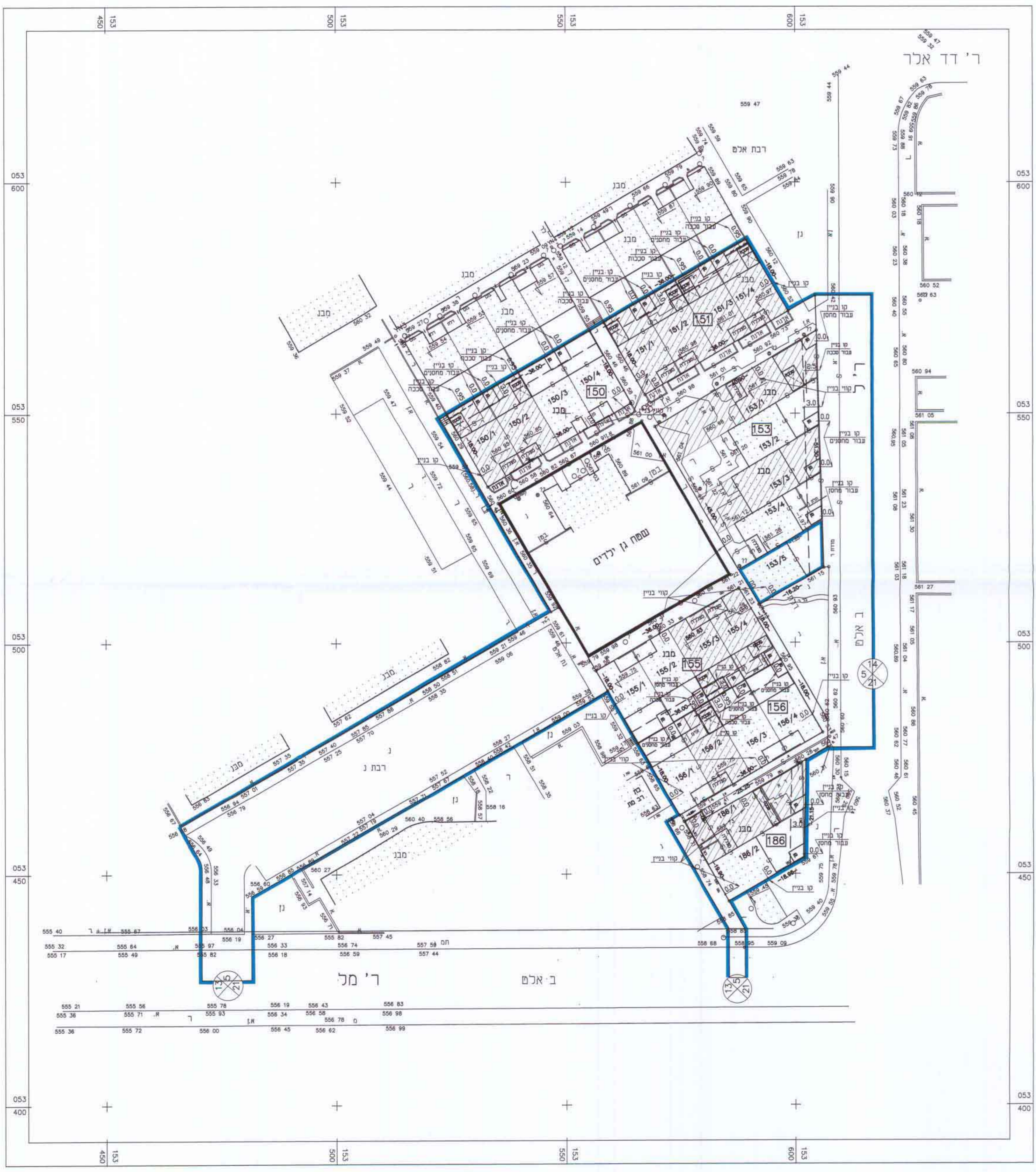
תכנית העמדה קני"מ 1:500
