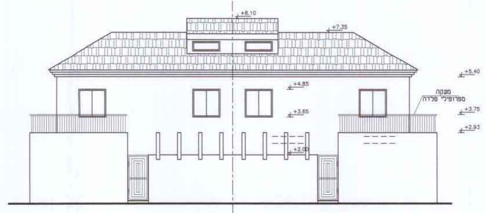
חזית קדמית קני"מ 1:100
