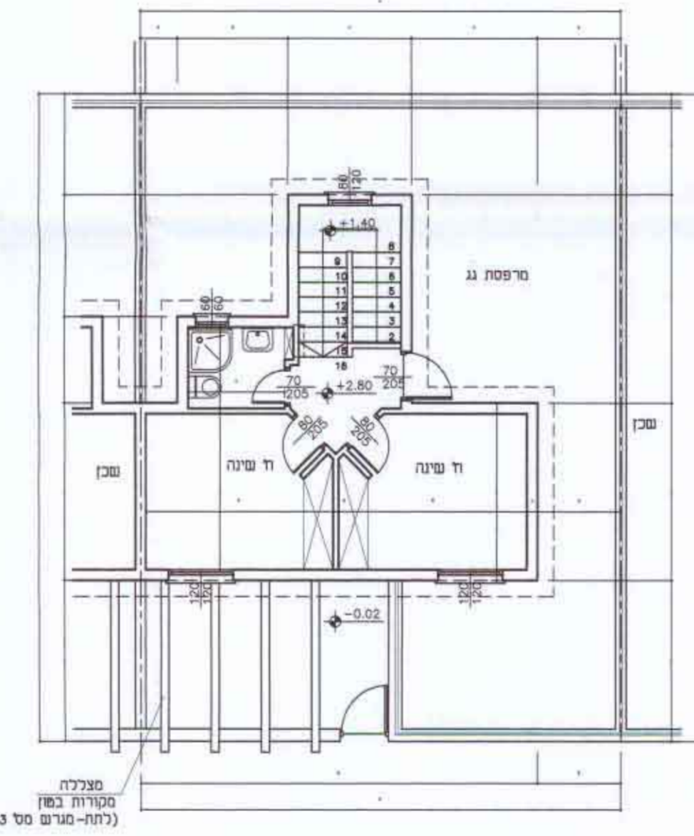
תכנית קומה א' קני"מ 1:100
