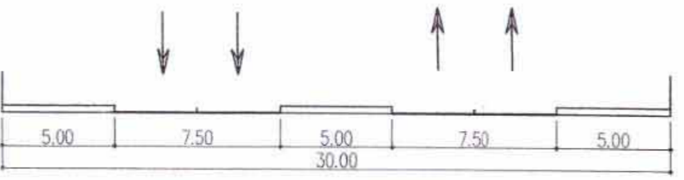
חתך 1-1
