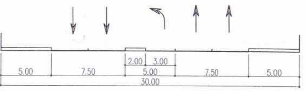
חתך 2-2
