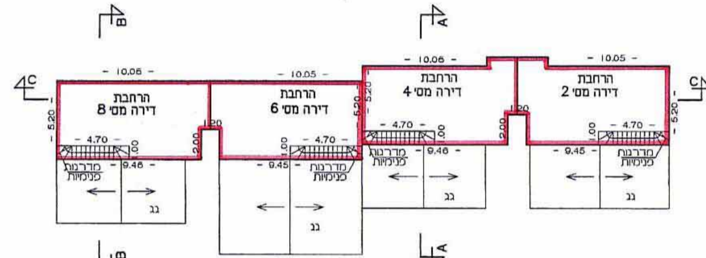
קומה ב' ק.מ. 1:250
