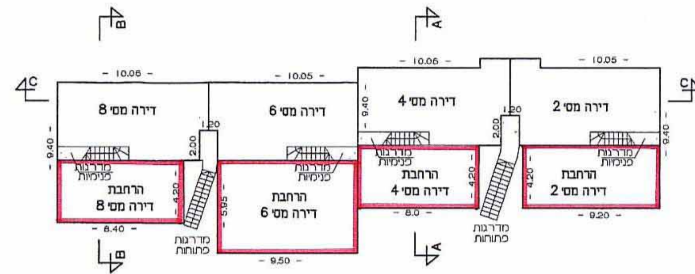
קומה א' ק.מ. 1:250
