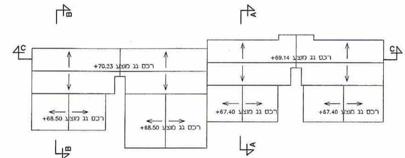
תכנית הגג ק.מ. 1:250
