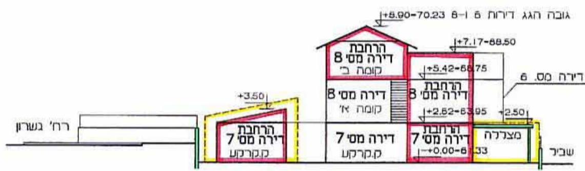
חתך B-B
