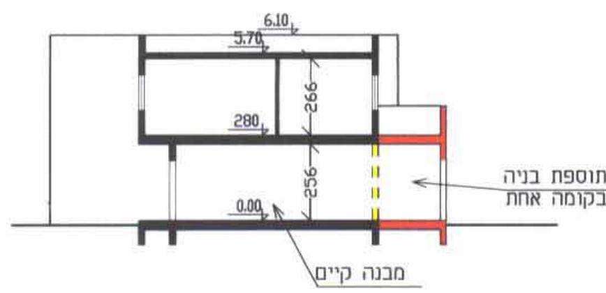
חלק א-א אופייני קנ"מ 1:200 עבור מגרשים מס' 264/2, 265/1
