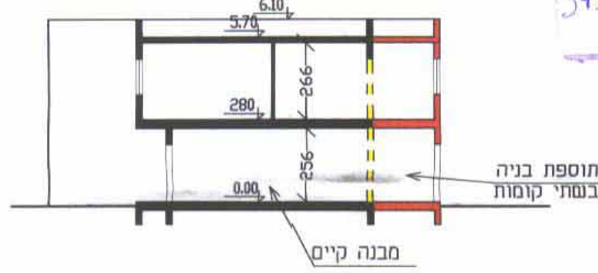
חלק א-א אופייני קנ"מ 1:200 עבור מגרש מס' 253/2
