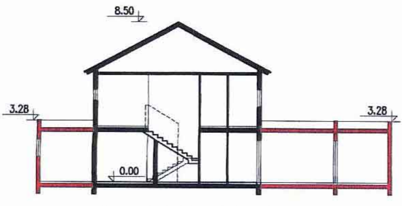
חתך א-א קנ"מ 1:200
