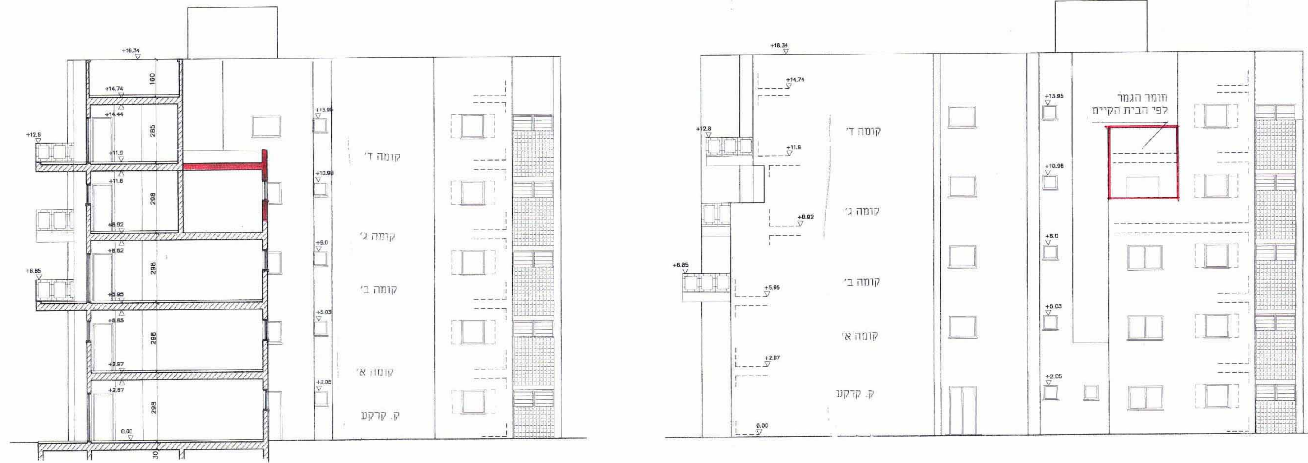
חזית צפון מזרחית ק"מ 1:100
