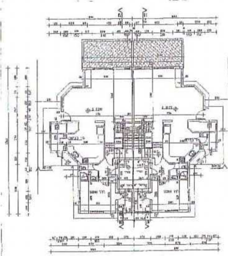
תכנית קומת קרקע מצב קיים למרצע 1:250
