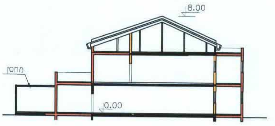
חתך א-א קנ"מ 1:200
