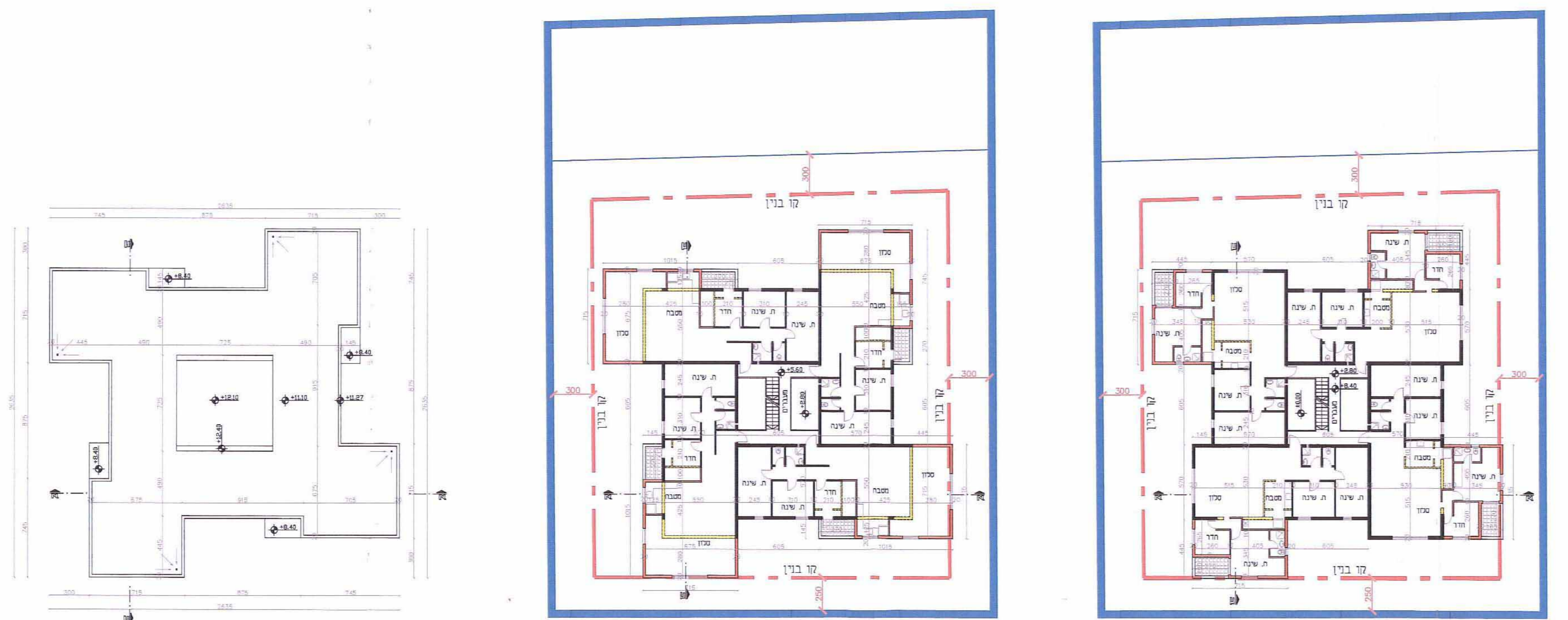
תכנית קומה א' קני"מ 1:200, תכנית קומה ב' קני"מ 1:200, תכנית קומה ג' קני"מ 1:200
