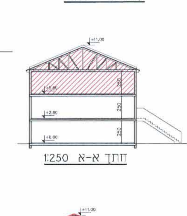
חית א-א 1:250
