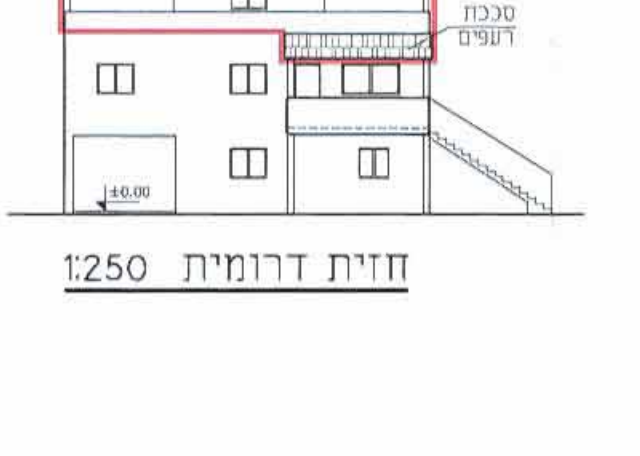
חזית דרומית 1:250
