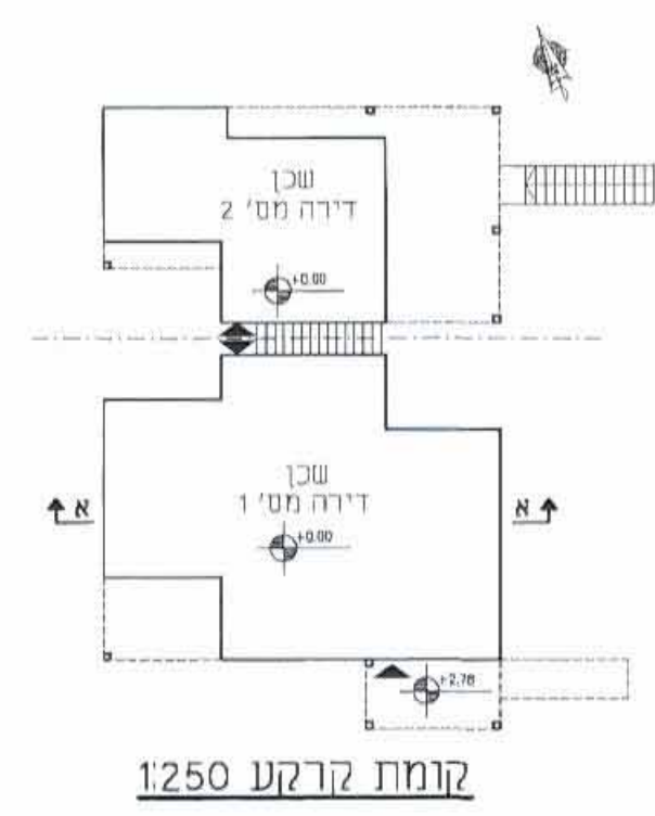
קומת קרקע 1:250
