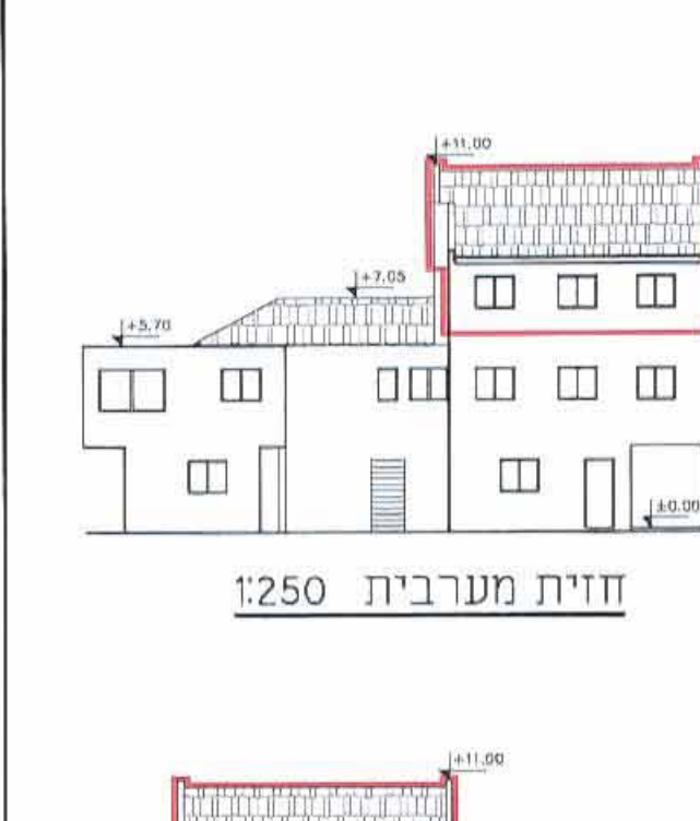
חזית מערבית 1:250
