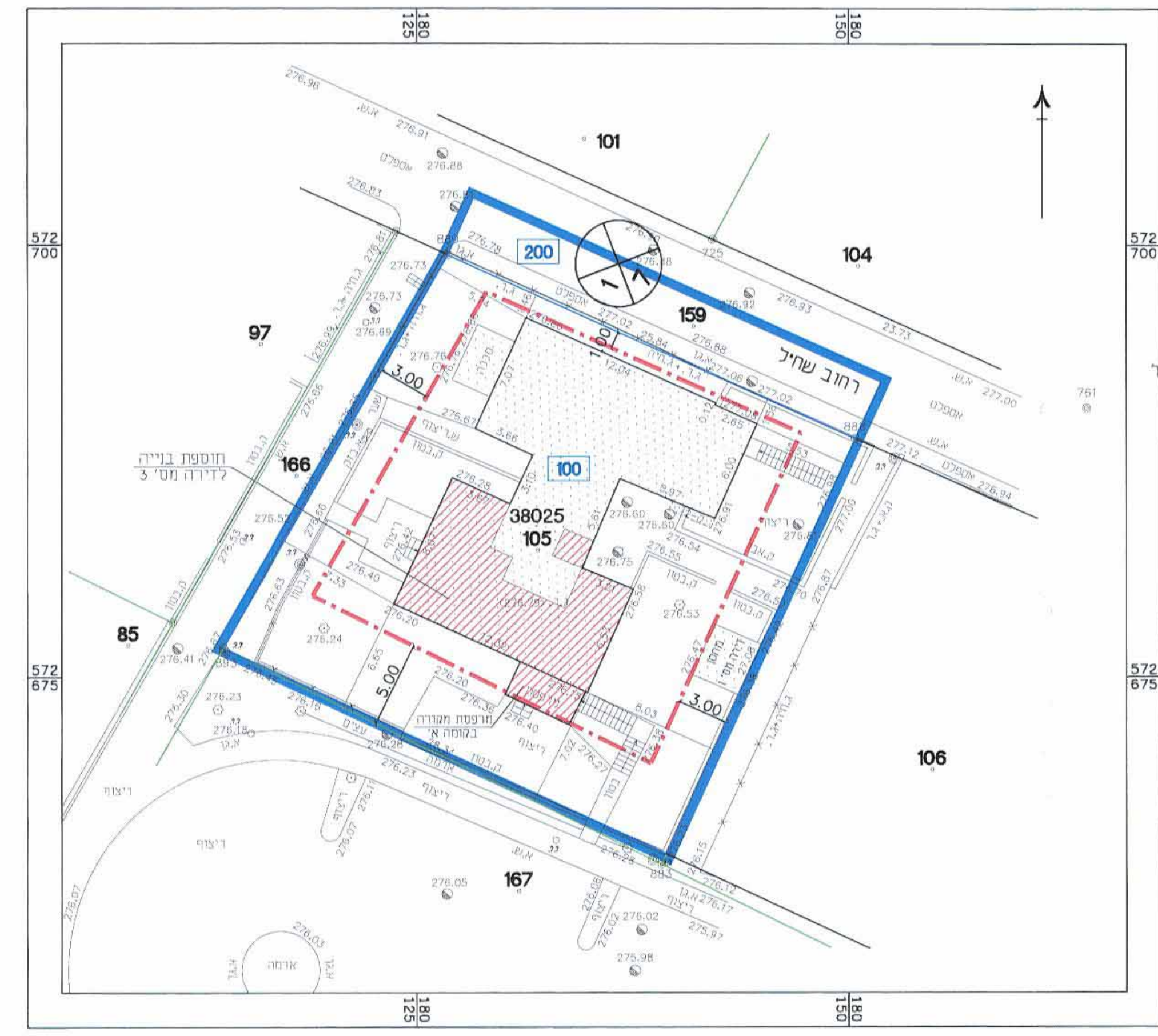
תרשים המגרש 1:250
