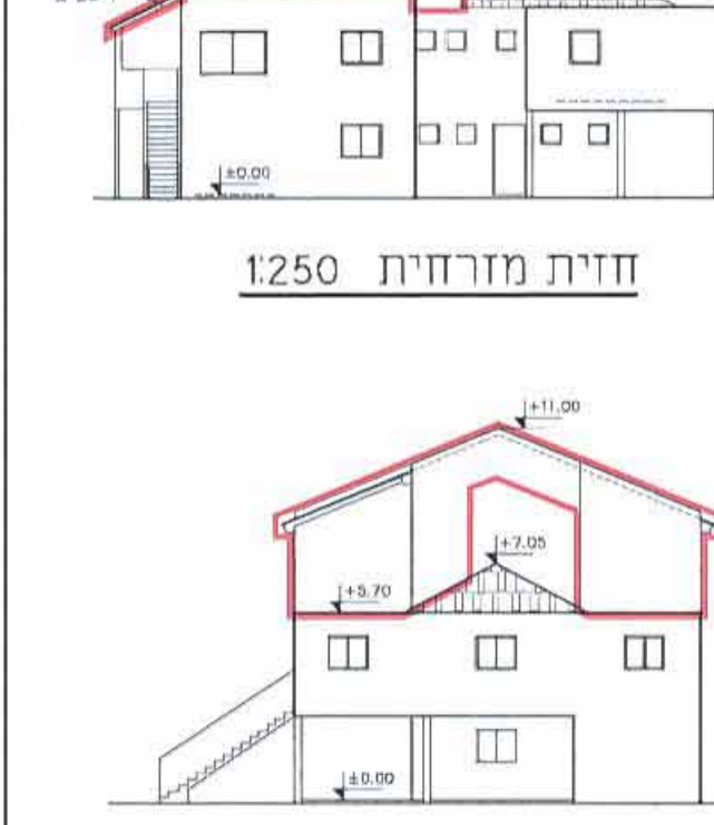
חזית מזרחית 1:250
