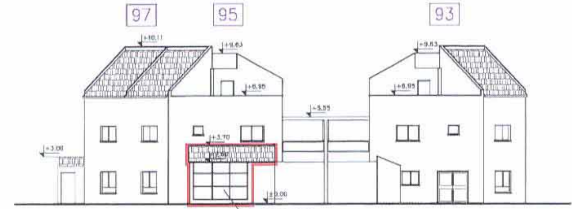
חזית מערבית 1:250
