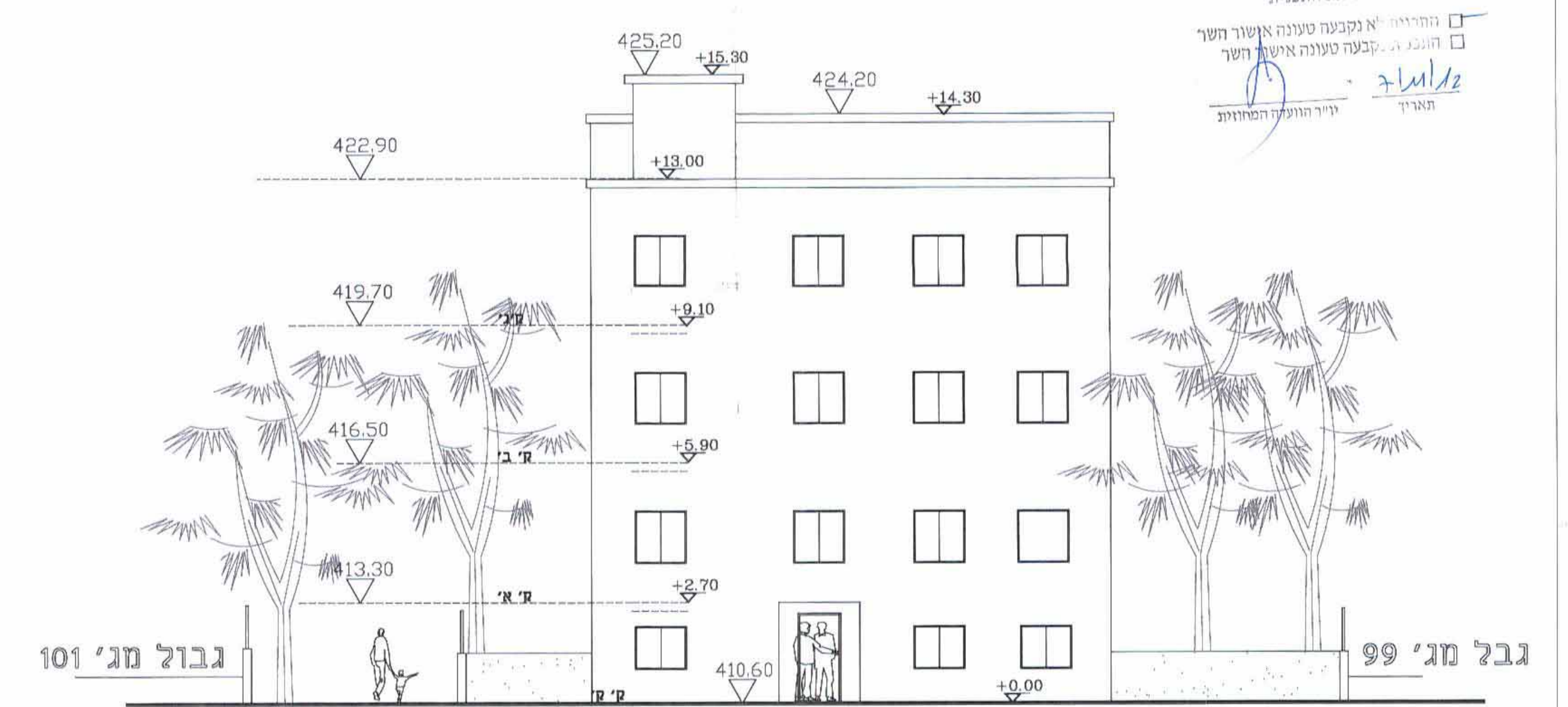
חזית קדמית מבנה מס' 2 ק.מ. 1:100
