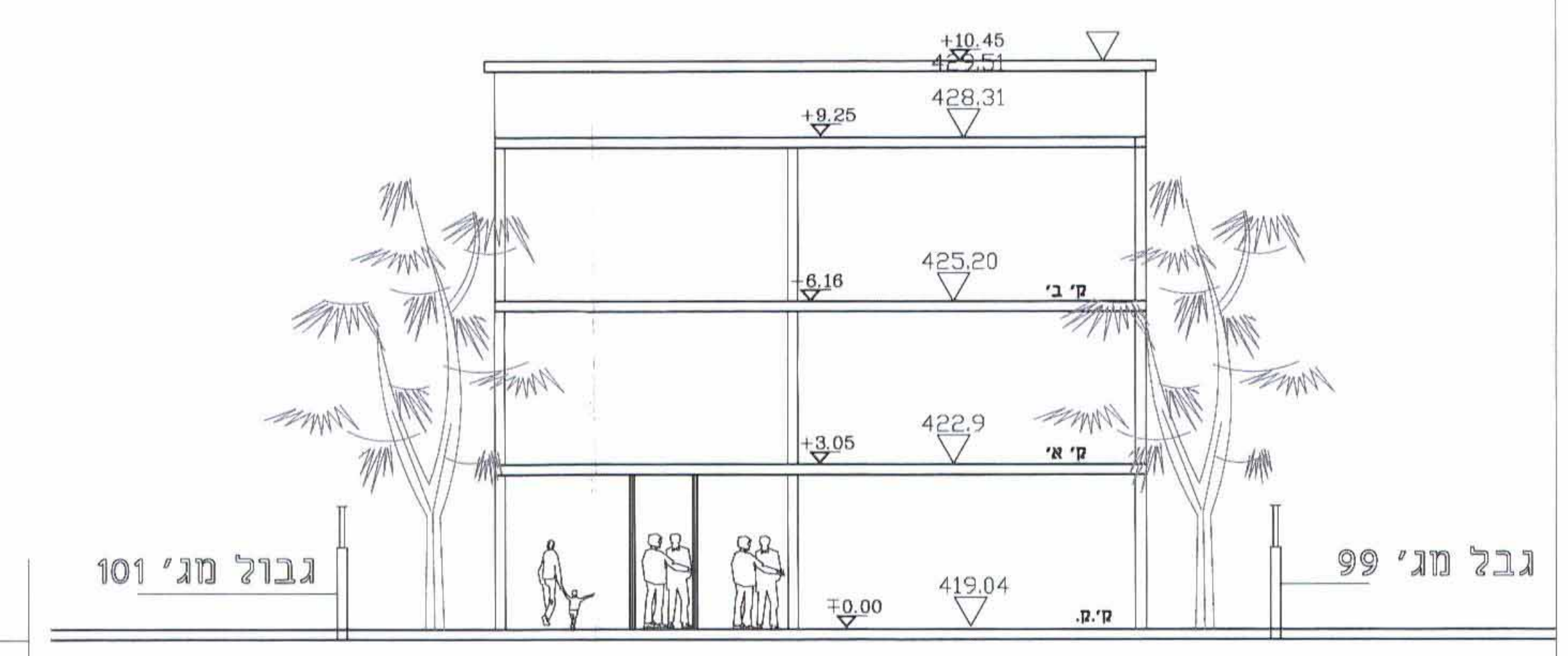
חזית קדמית מבנה מס' 2 ק.מ. 1:100
