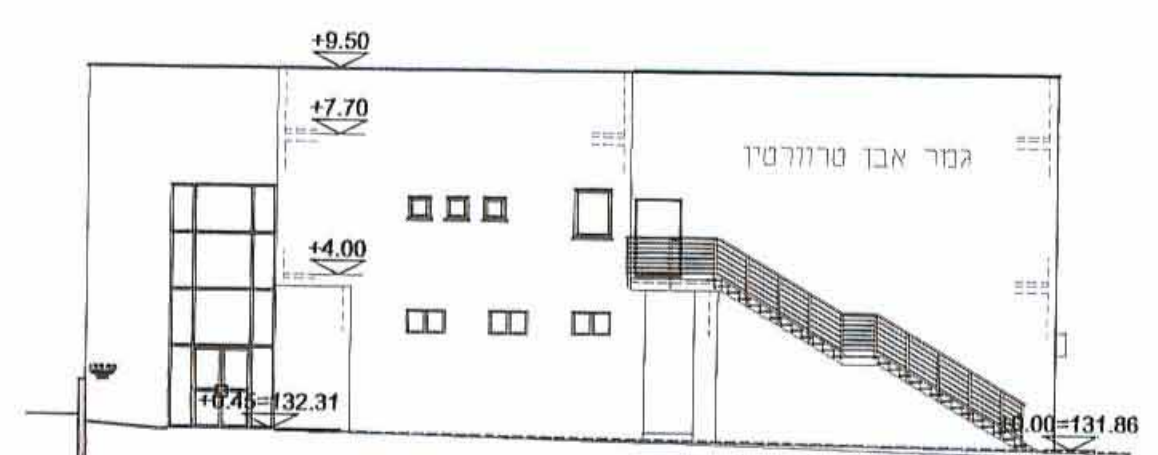
חזית לחנייה קני"מ 200:1
