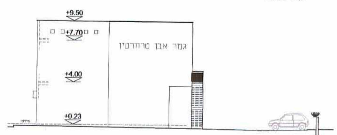
חזית לשכן קני"מ 200:1
