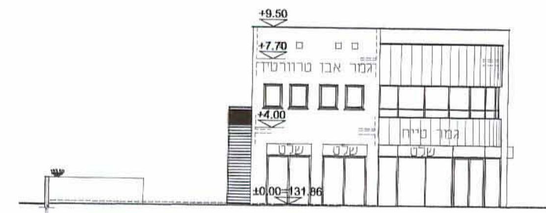
חזית לרחוב תותחנים קני"מ 200:1
