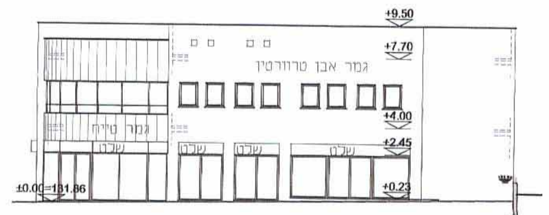
חזית לרחוב חיל הנדסה קני"מ 200:1
