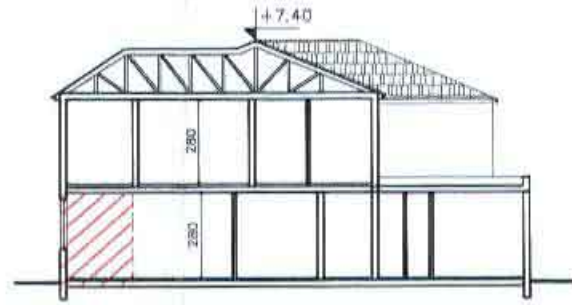
חתך ב-ב 1:250
