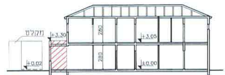
חתך א-א 1:250
