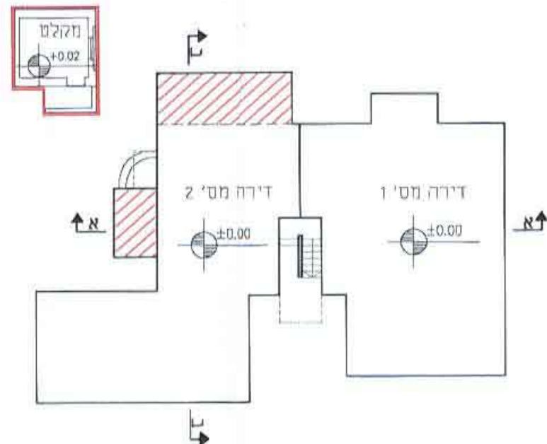
קומת קרקע 1:250
