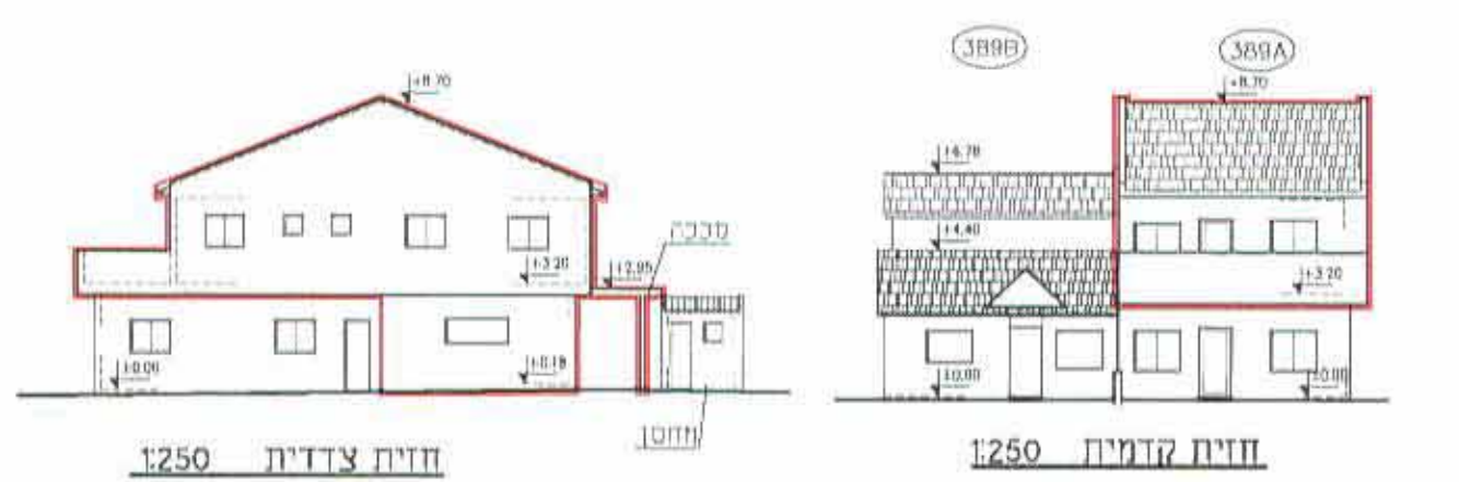
חיתך א-א 1:250 חיתך ב-ב 1:250
