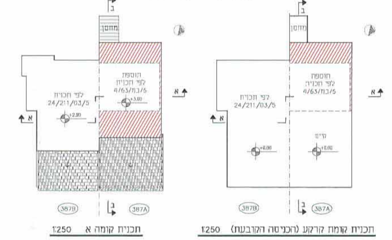
תכנית קומת קרקע (הכניסה הקובעת) 1:250 תכנית קומה א 1:250
