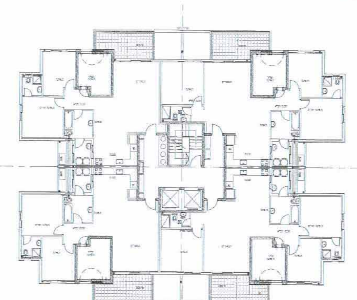
תכנית קומה סיפוסית קנ"מ 1:200
