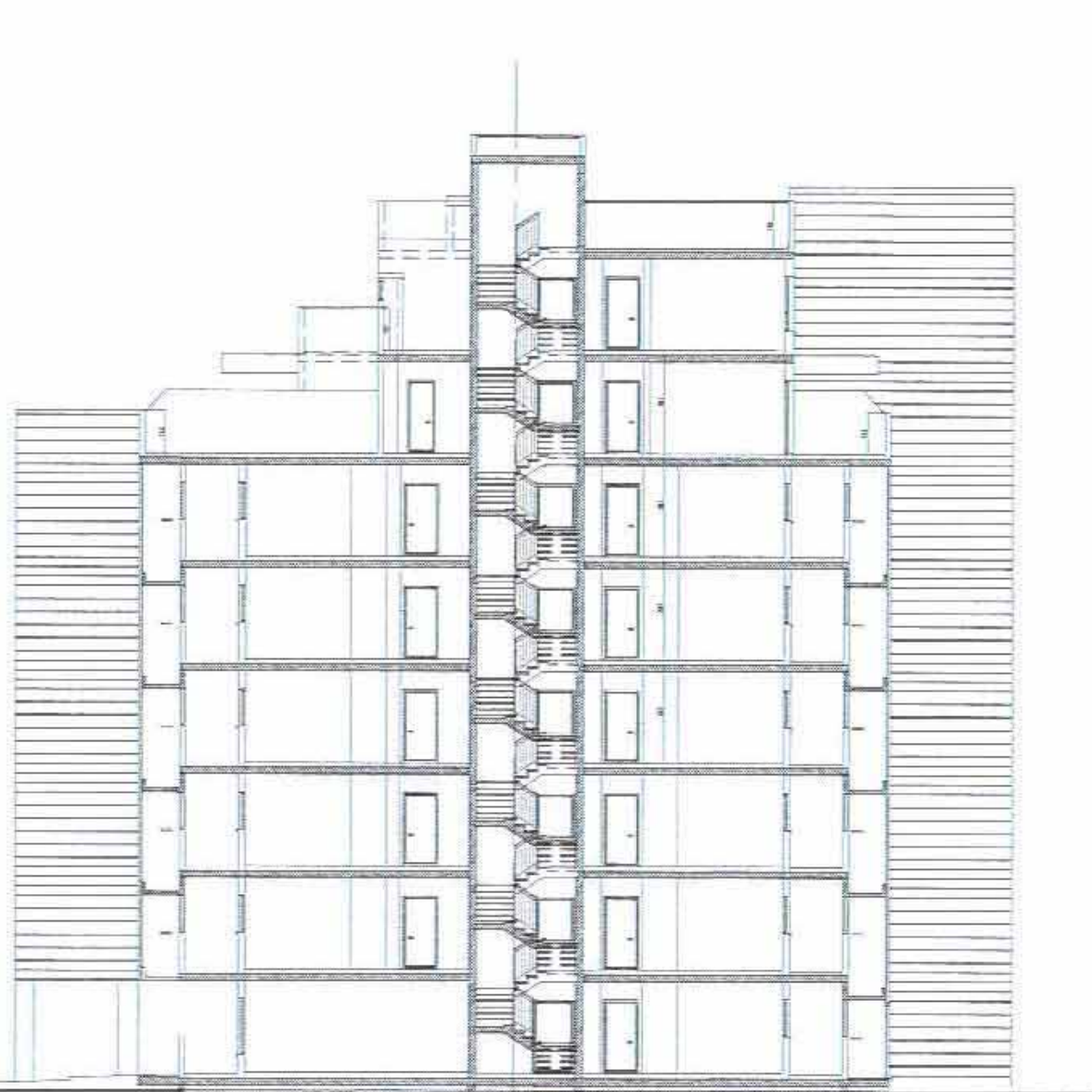
חתך ב-ב קנ"מ 1:200
