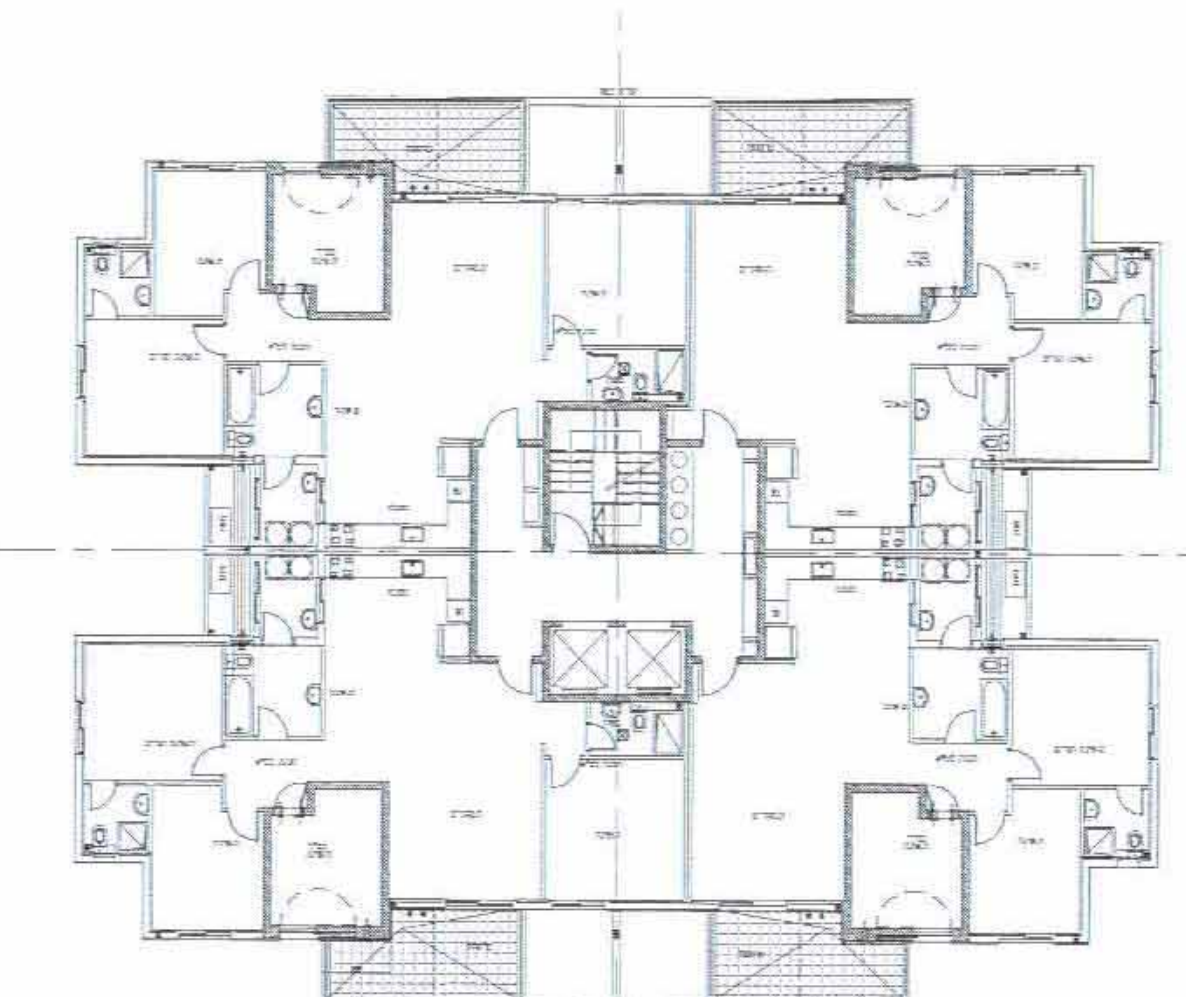
תכנית קומה טיפוסית קנ"מ 1:200
