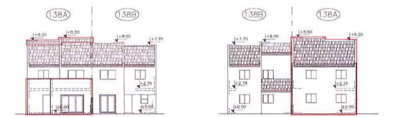
חזית קדמית 1:250 חזית לרחוב אציל 1:250
