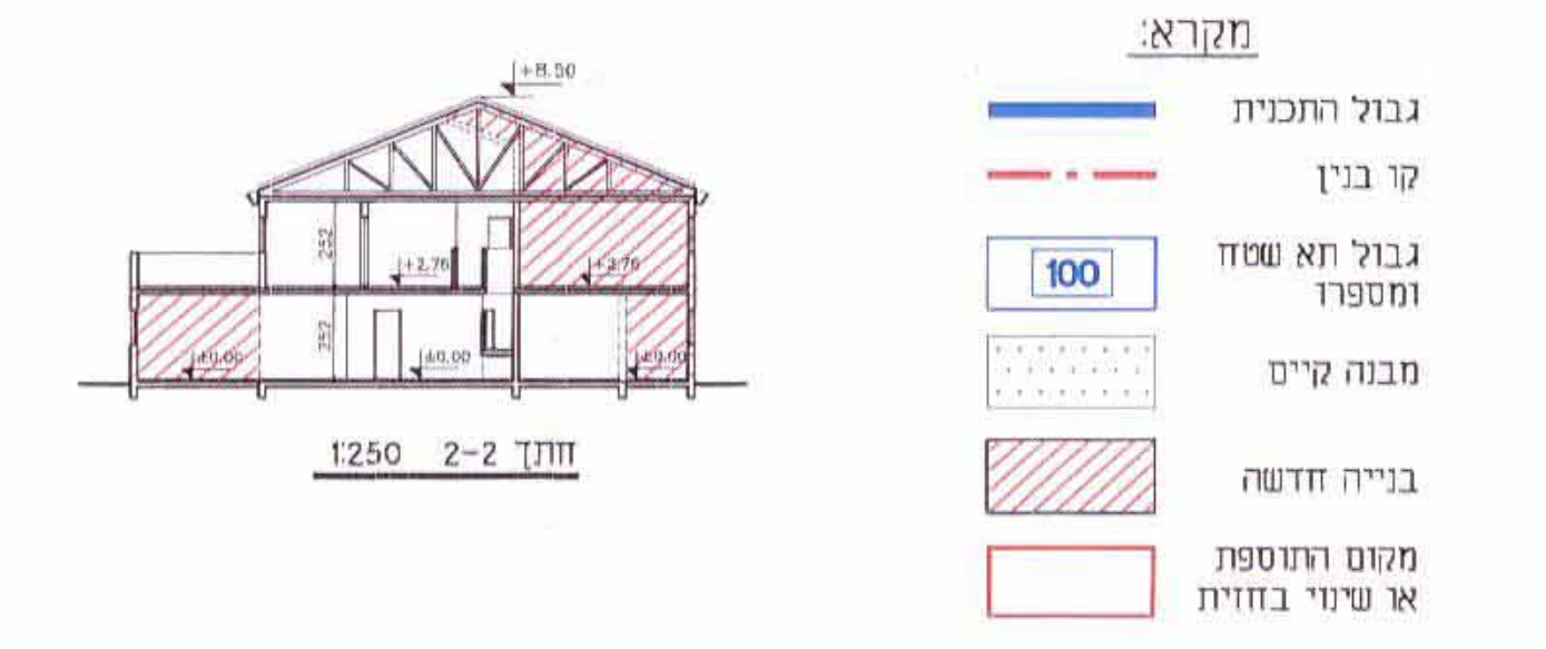
חזית 2-2 1:250
