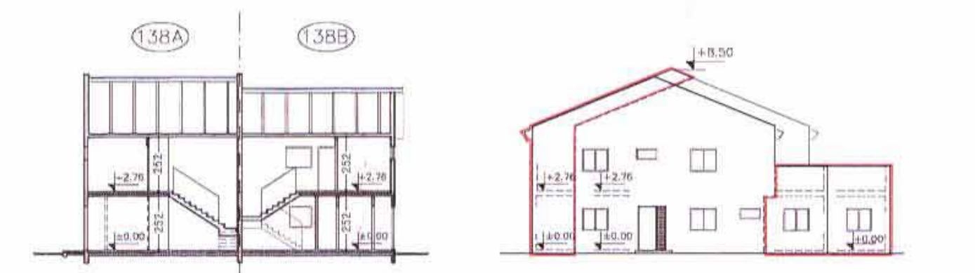
חזית צדדית 1:250 חזית צדדית 1:250
