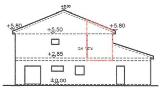
חית צדית 1:250
