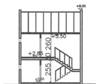
חתך 1-1 1:250
