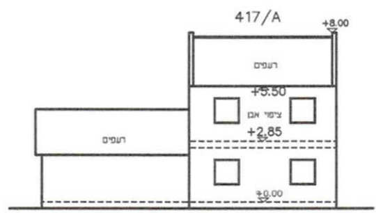
חית אחורית 1:250
