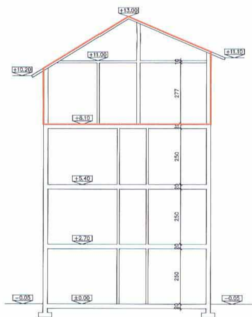
חתך ב-ב ק"מ 1:100
