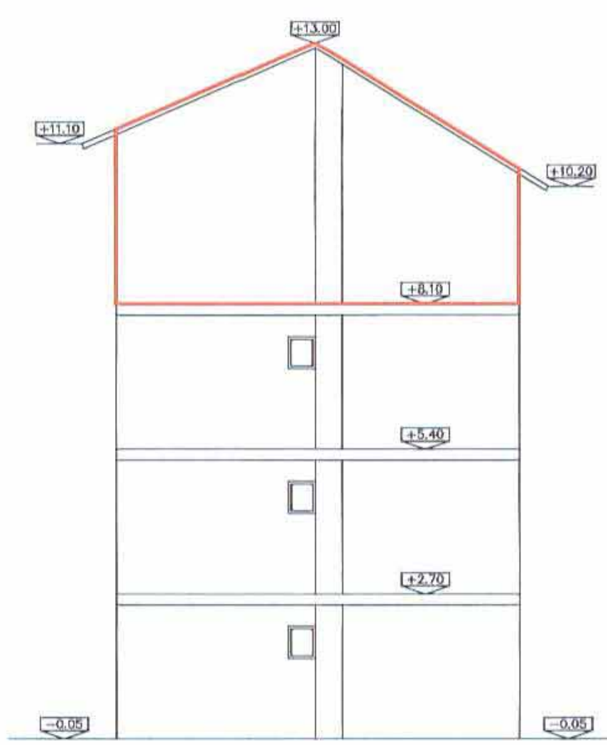
חזית צדדית ק"מ 1:100
