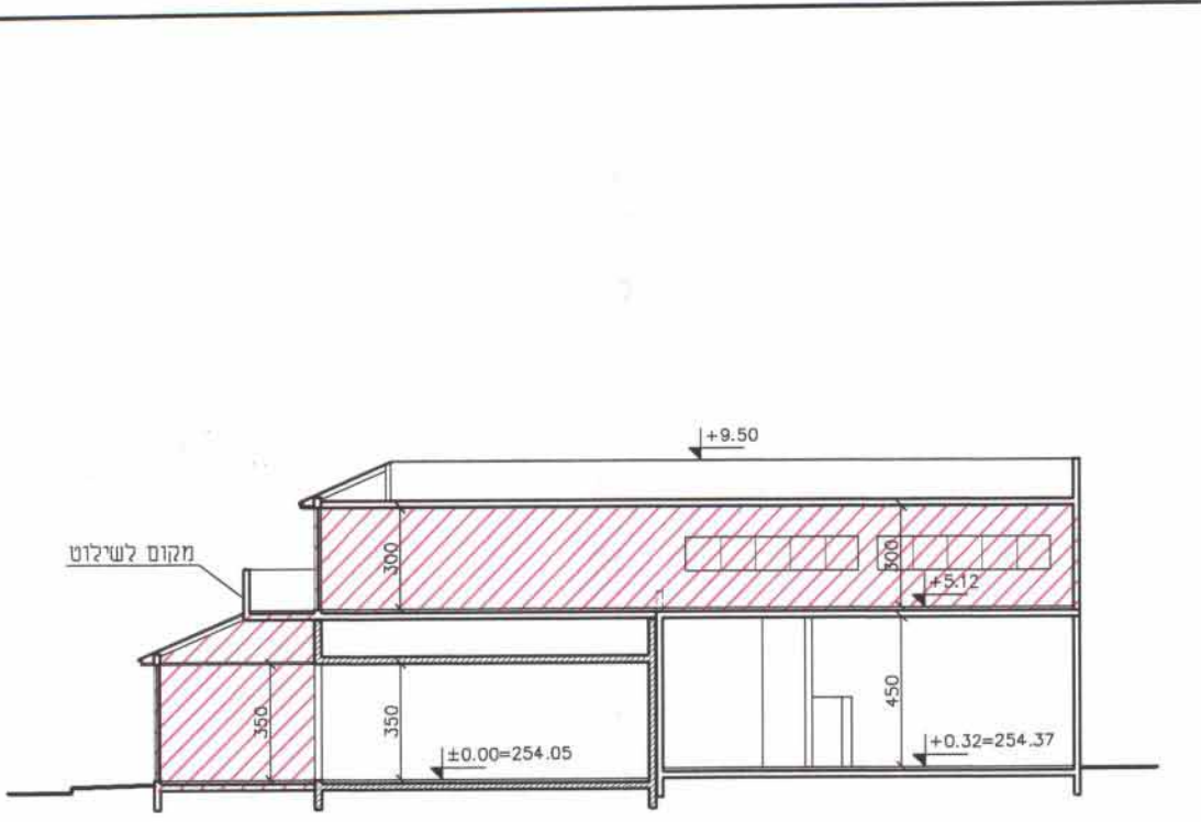
חתך ב-ב 1:250
