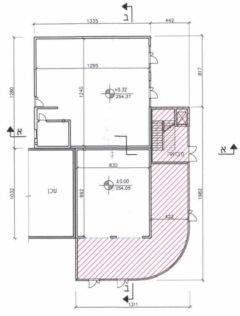
תכנית קומת קרקע 1:250
