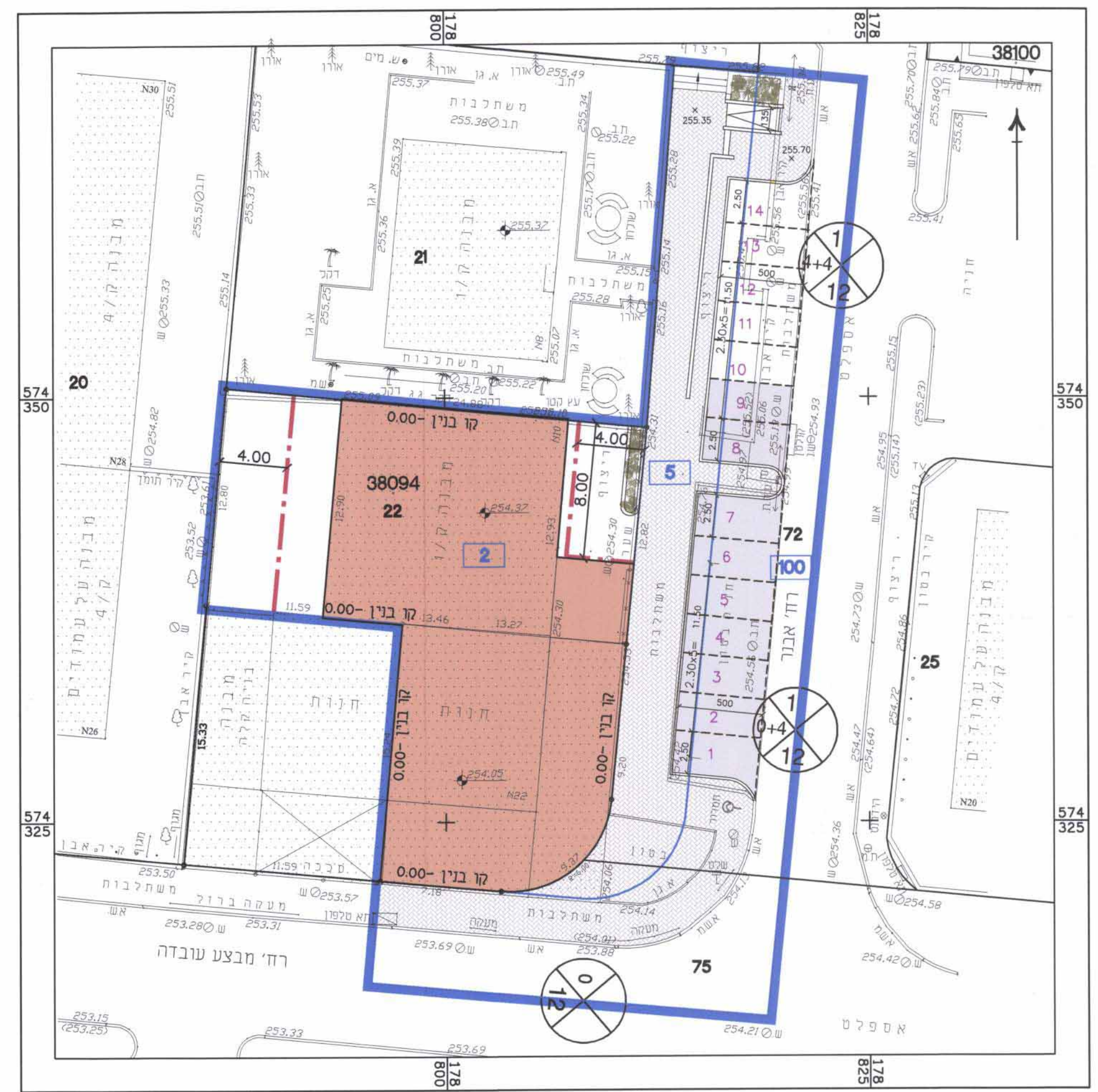
תכנית העמדה 1:250
