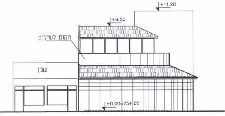
חתך צ-צ 1:250
