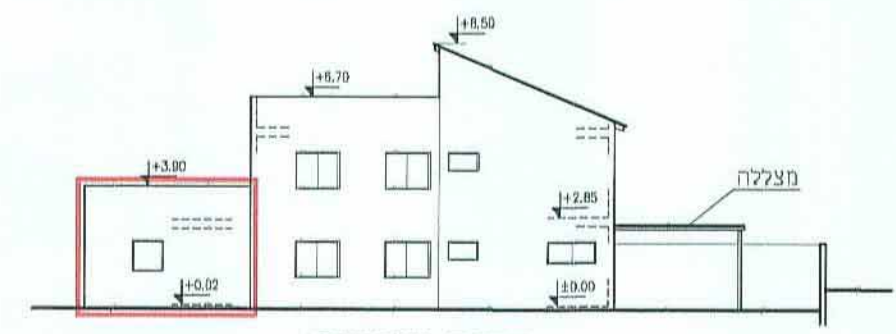
חזית צדדית 1:250
