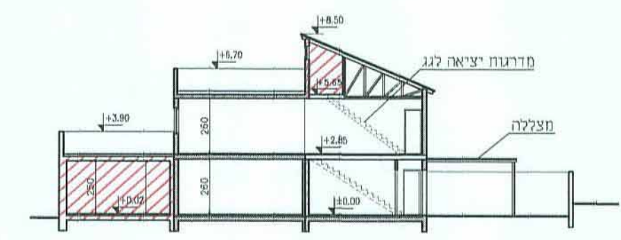
חתך א-א 1:250
