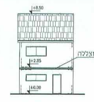
חזית קדמית 1:250
