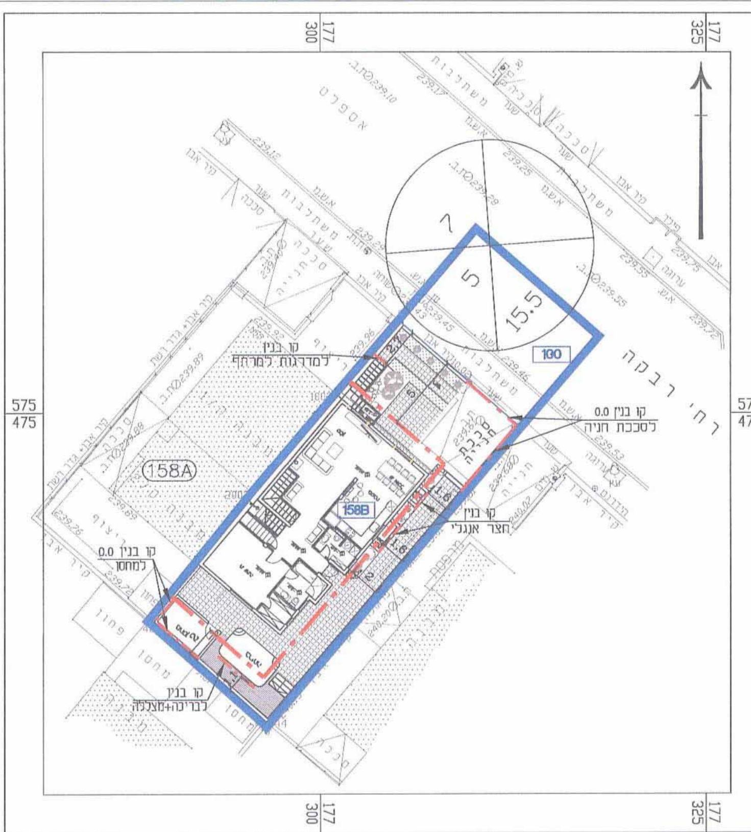
תכנית העמדה ופיתוח ק.מ. 1:250
