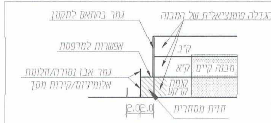
③ תכנית בינוי להרחבת מבנה הכוללת חזית מסחרית במבנה קיים חלופה א' - המבנה הקיים לא חורג מקווי הבנין
