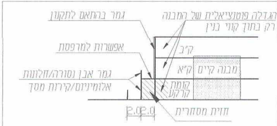
④ תכנית בינוי להרחבת מבנה הכוללת חזית מסחרית במבנה קיים חלופה ב' - המבנה הקיים חורג מקווי הבנין
