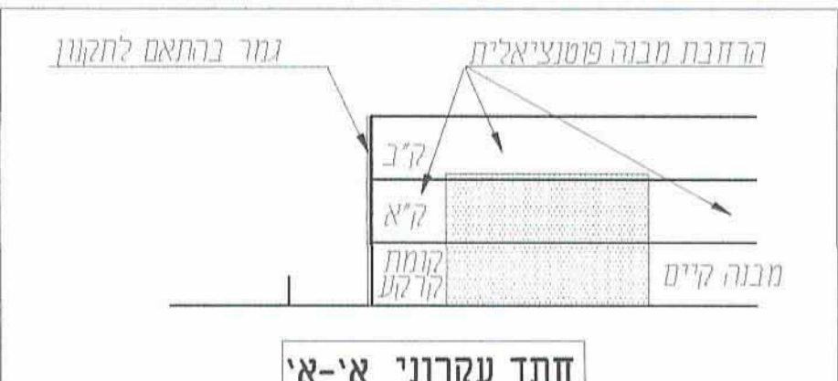
⑤ תכנית בינוי להרחבת מבנה קיים חלופה א' - המבנה הקיים לא חורג מקווי הבנין
