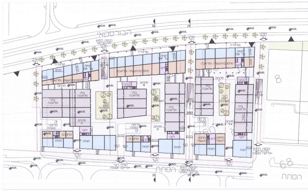
תכנית בינוי - מתחם הבורסקאי - מפלס הקרקע גר"מ 1:500
