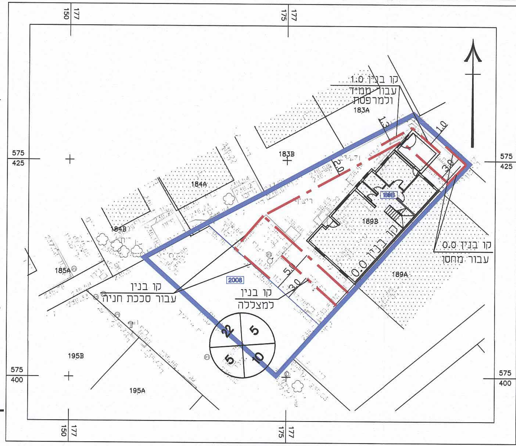
תרשים המגרש קנה מידה 1:250
