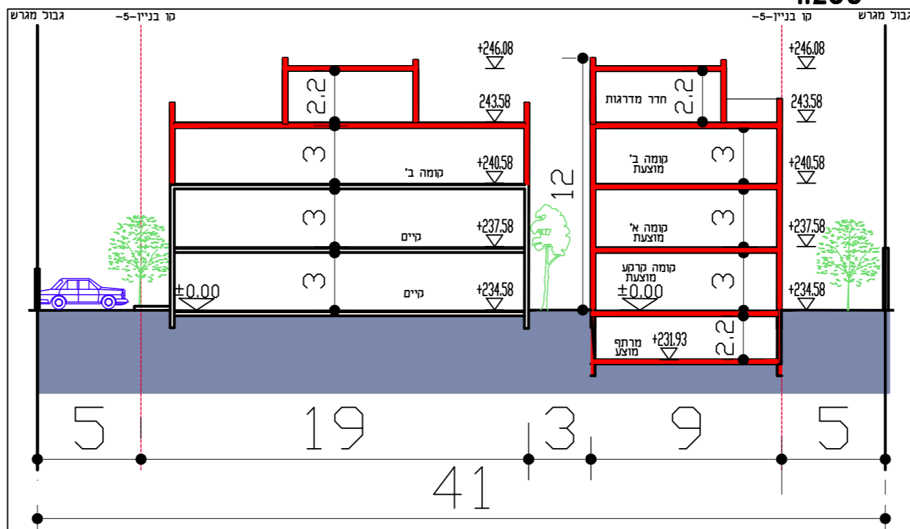
חתך טיפוסי A-A 1:250
