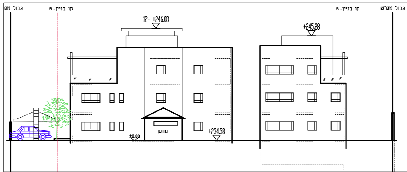
חזית 1:250
