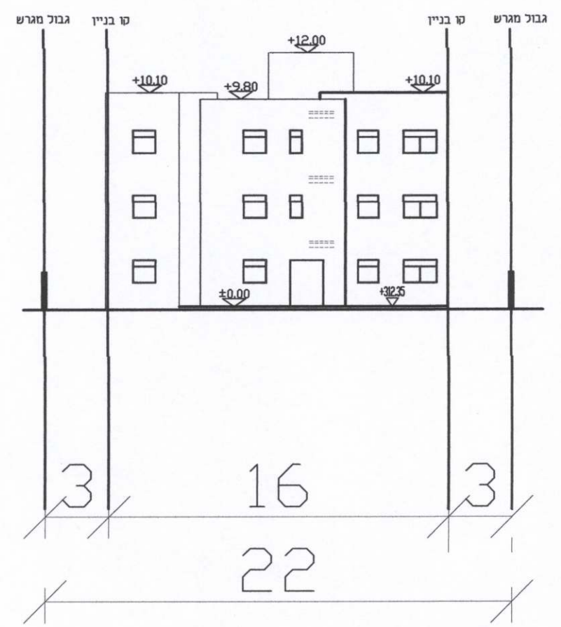
חזית רחוב 1:250
