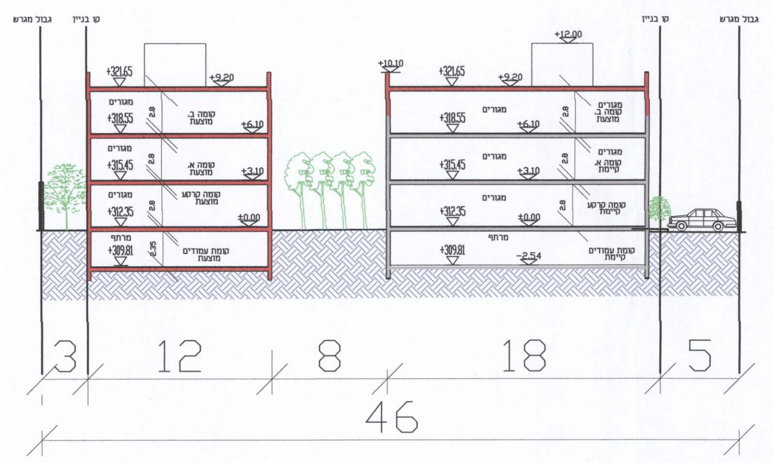
חתך טיפוסי 1:250 A-A
