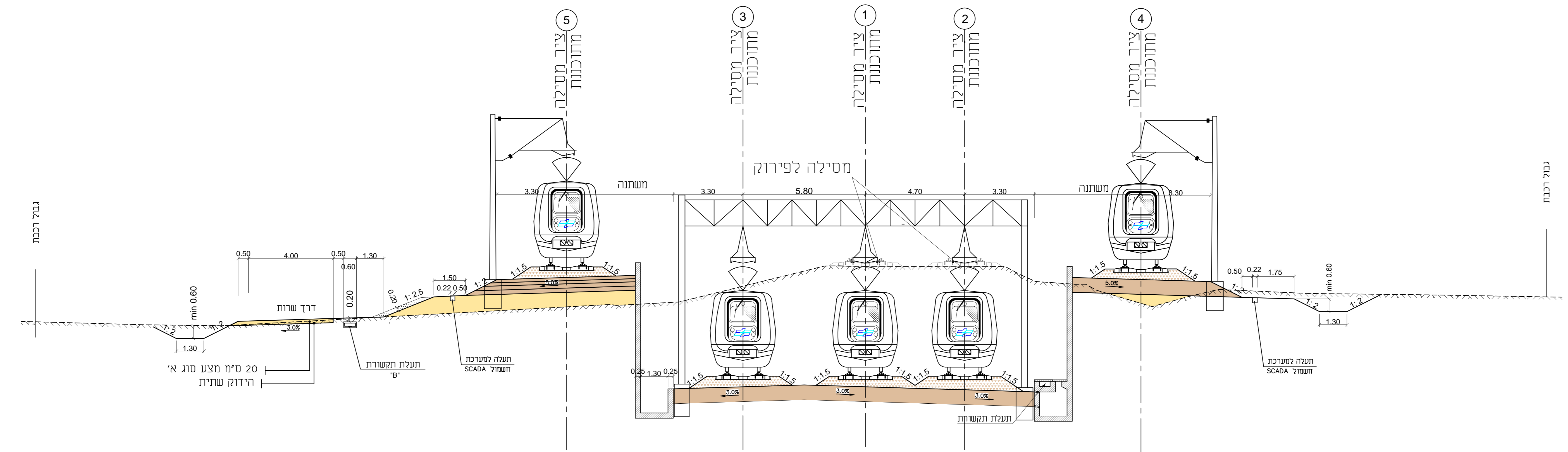
חתך טיפוסי באזור נחל סוללים ק"מ 6+325-6+675
