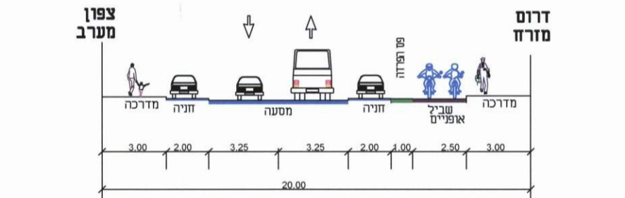
כביש מסי 6 קטע כביש 5 - כביש 73 ברוחב 20.00 מ'
