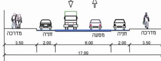
כביש מסי 7 ברוחב 17.00 מ' קטע פנימי
