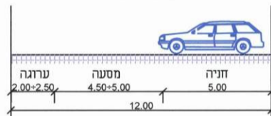
רחוב משולב ברוחב 12.00 מ'
