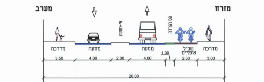
רחוב מסי 8 קטע מזרחי ברוחב 20.00 מ'
