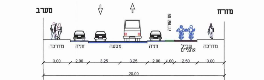
כביש מסי 6 קטע כביש 5 - כביש 73 ברוחב 20.00 מ'
