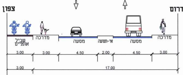
כביש מסי 9 ברוחב 17.00 מ'
