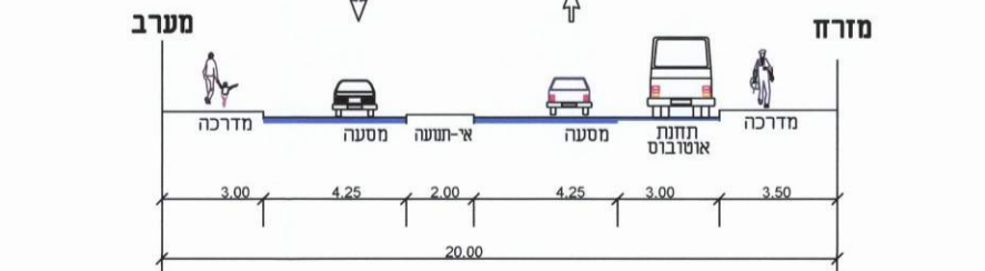
כביש מסי 8 ברוחב 20.00 מ'
