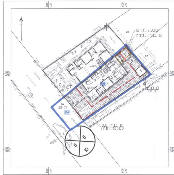
תכנית מגרש קני"מ 1:250
