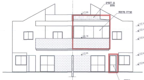
חזית קדמית קני"מ 1:100
