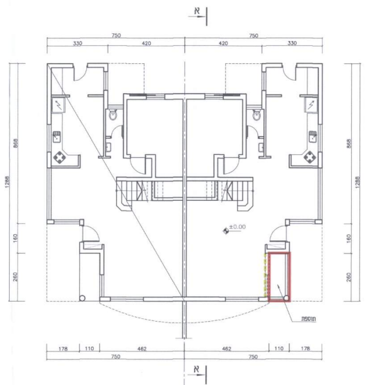
תכנית קומת קרקע קני"מ 1:100
