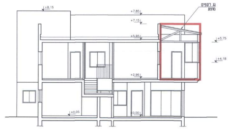
חלק א-א קני"מ 1:100
