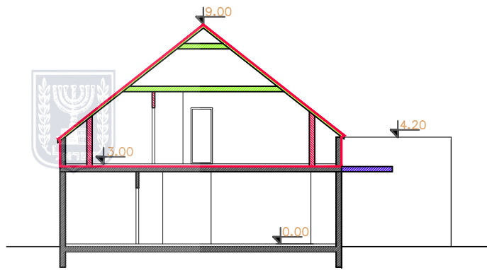
זו"ת א-א-קנ"מ 1 : 200
