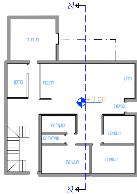
תכנית קומת גרעק קנ"מ 1 : 200
