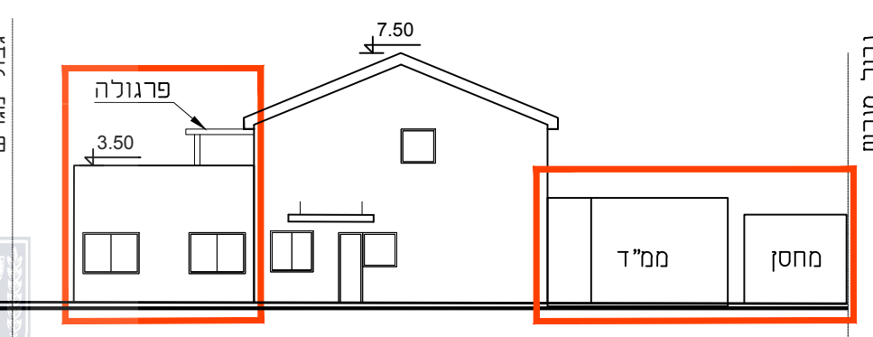
חזית צדדי קנ"מ 1:200
