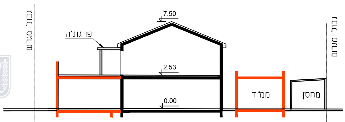
חתך א-א קנ"מ 1:200
