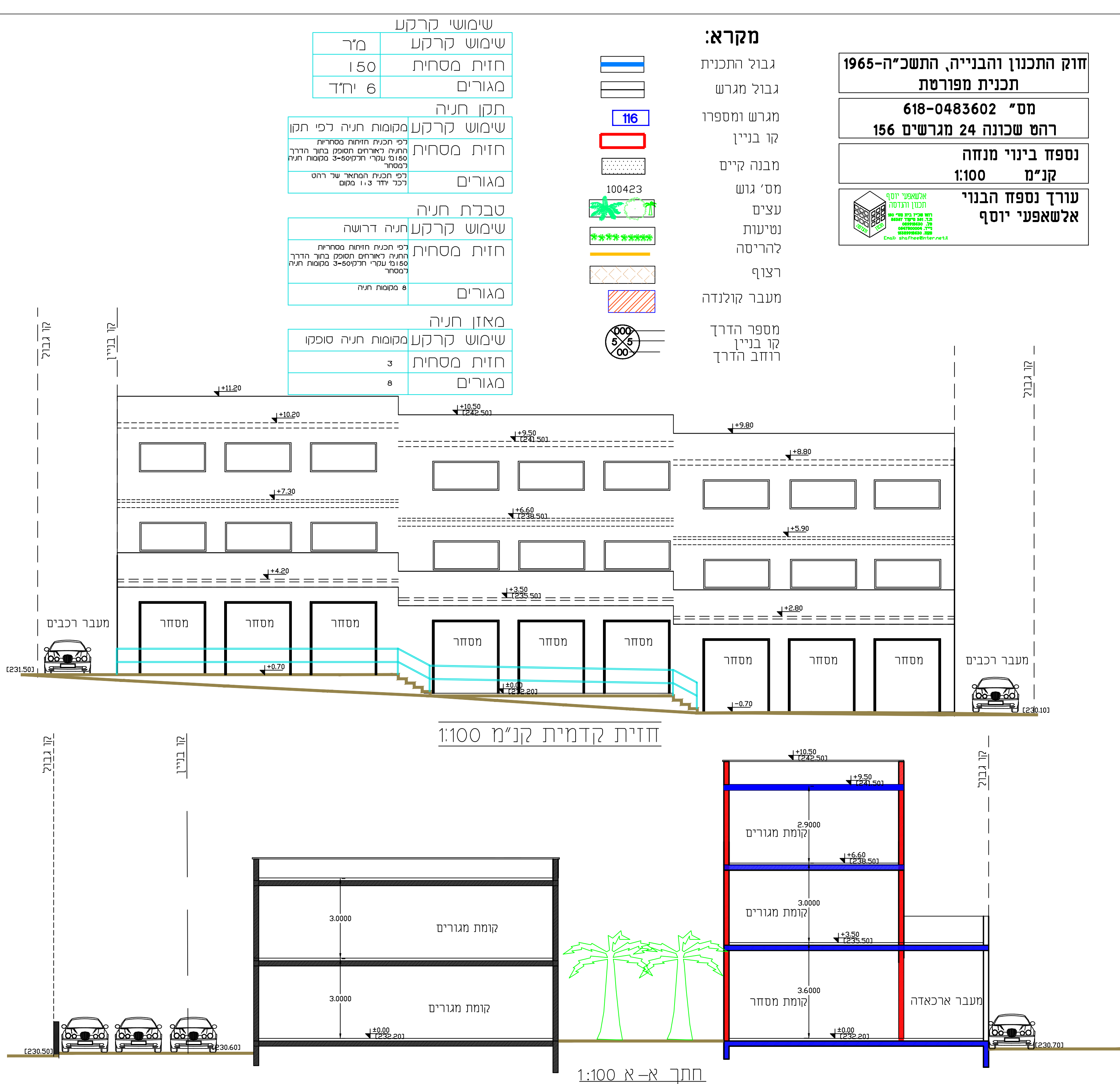
תכנית בנוי סכימטית למגרש 156 בשכונה 24 רהט 1:100
