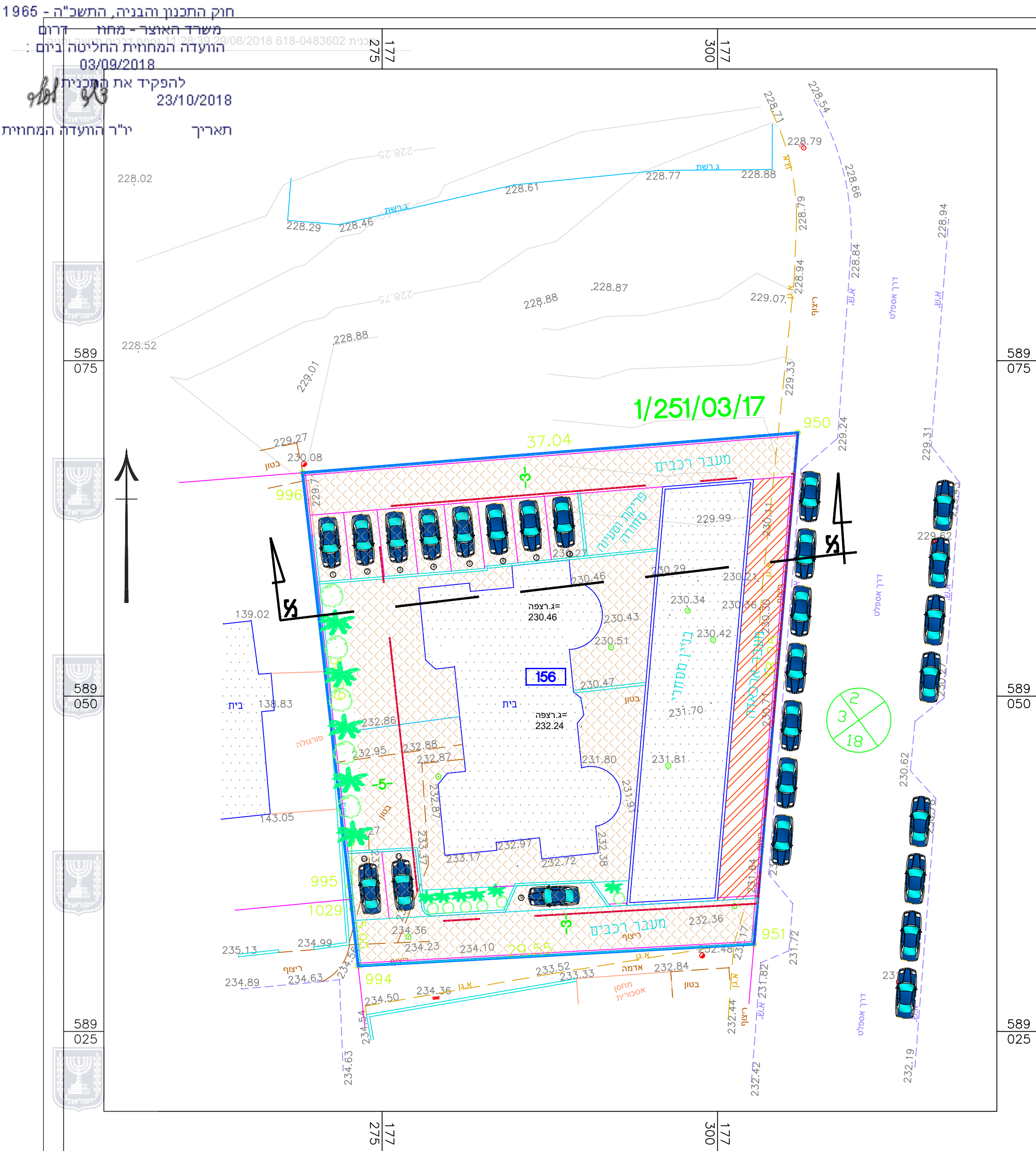
תכנית בנוי סכימטית למגרש 156 בשכונה 24 רהט 1:100
