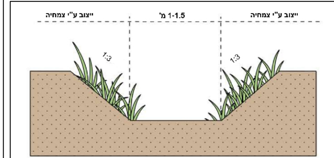
* פרט עקרוני לתעלות ניקוז מיוצבות בצמחיה
