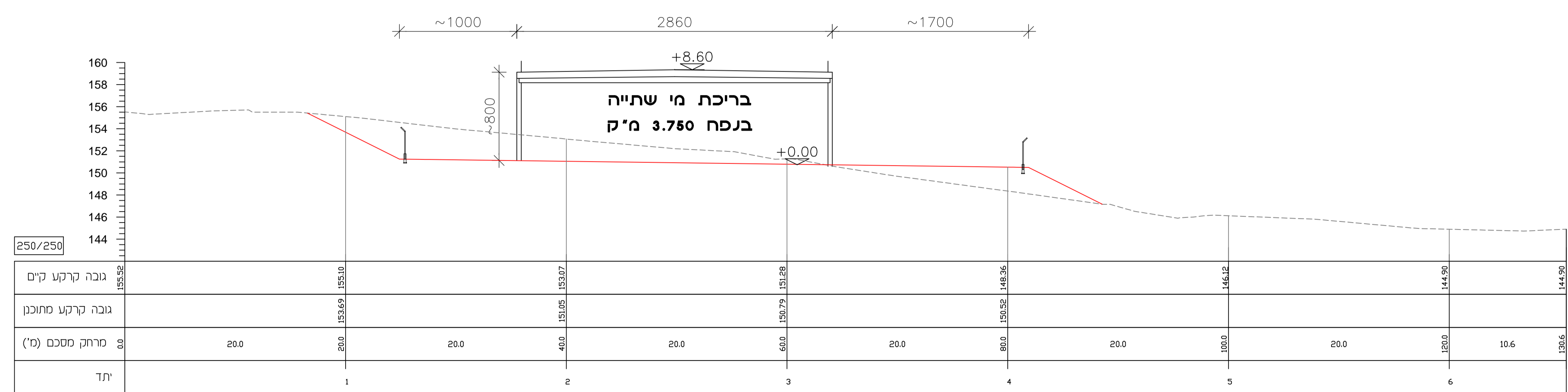
חתר ג'-ג' ±0.00=+151.25
