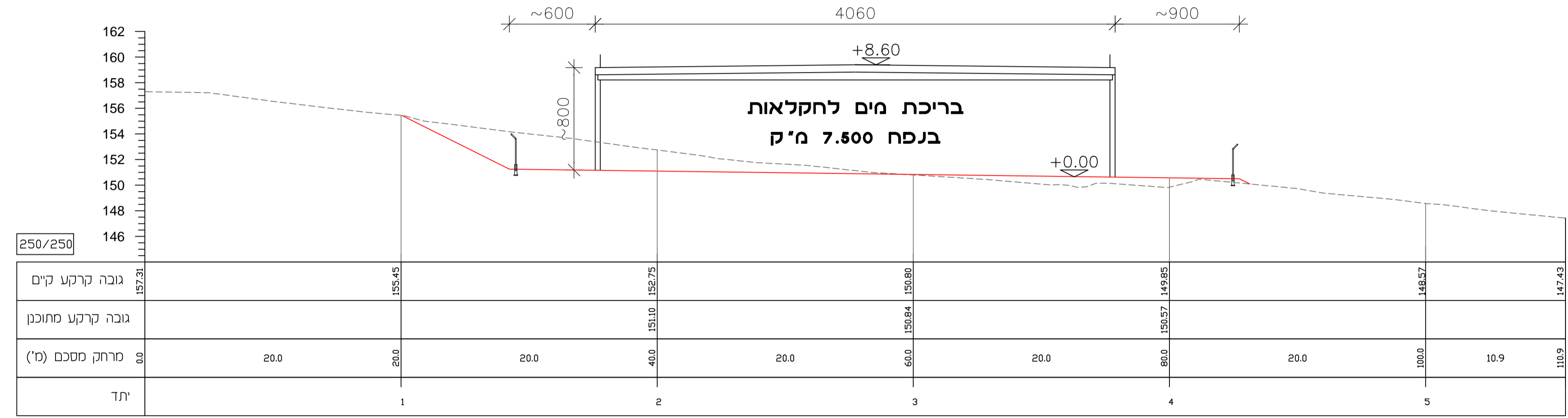
חתר ב'-ב' ±0.00=+151.25
