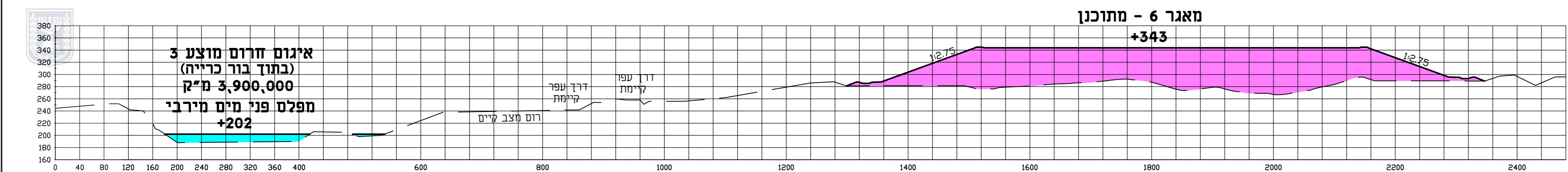
חתך ב-ב
