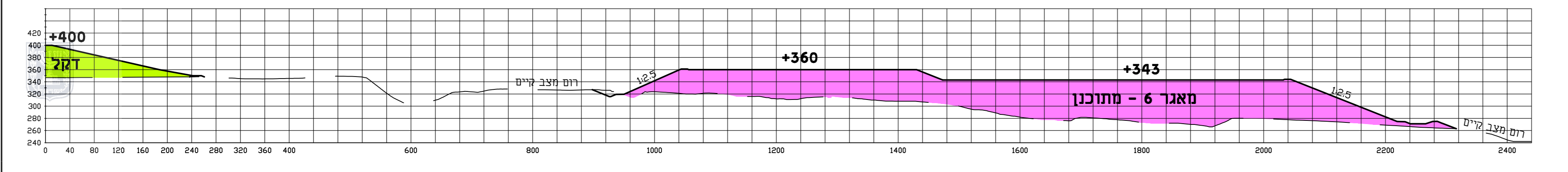
חתך ד-ד
