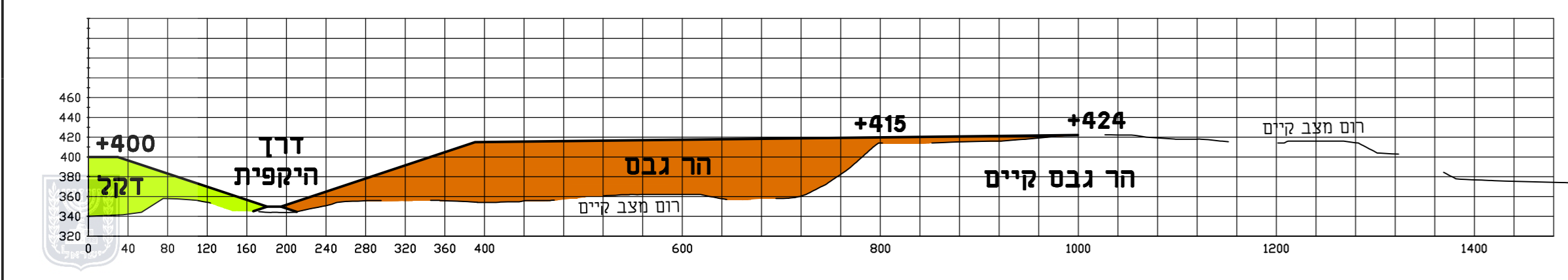
חתך ג-ג
