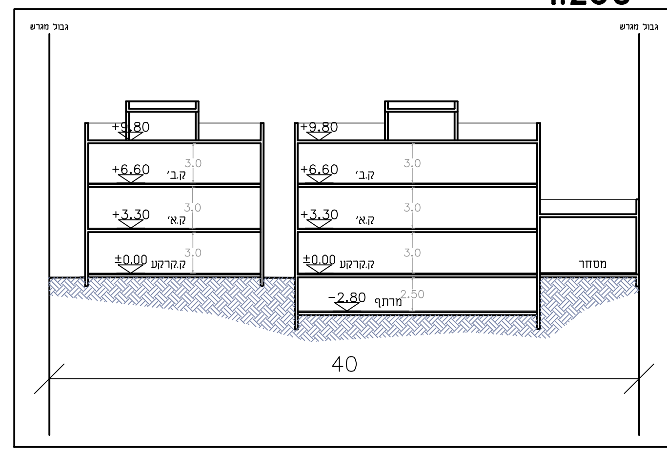
חתך טיפוסי A-A 1:250
