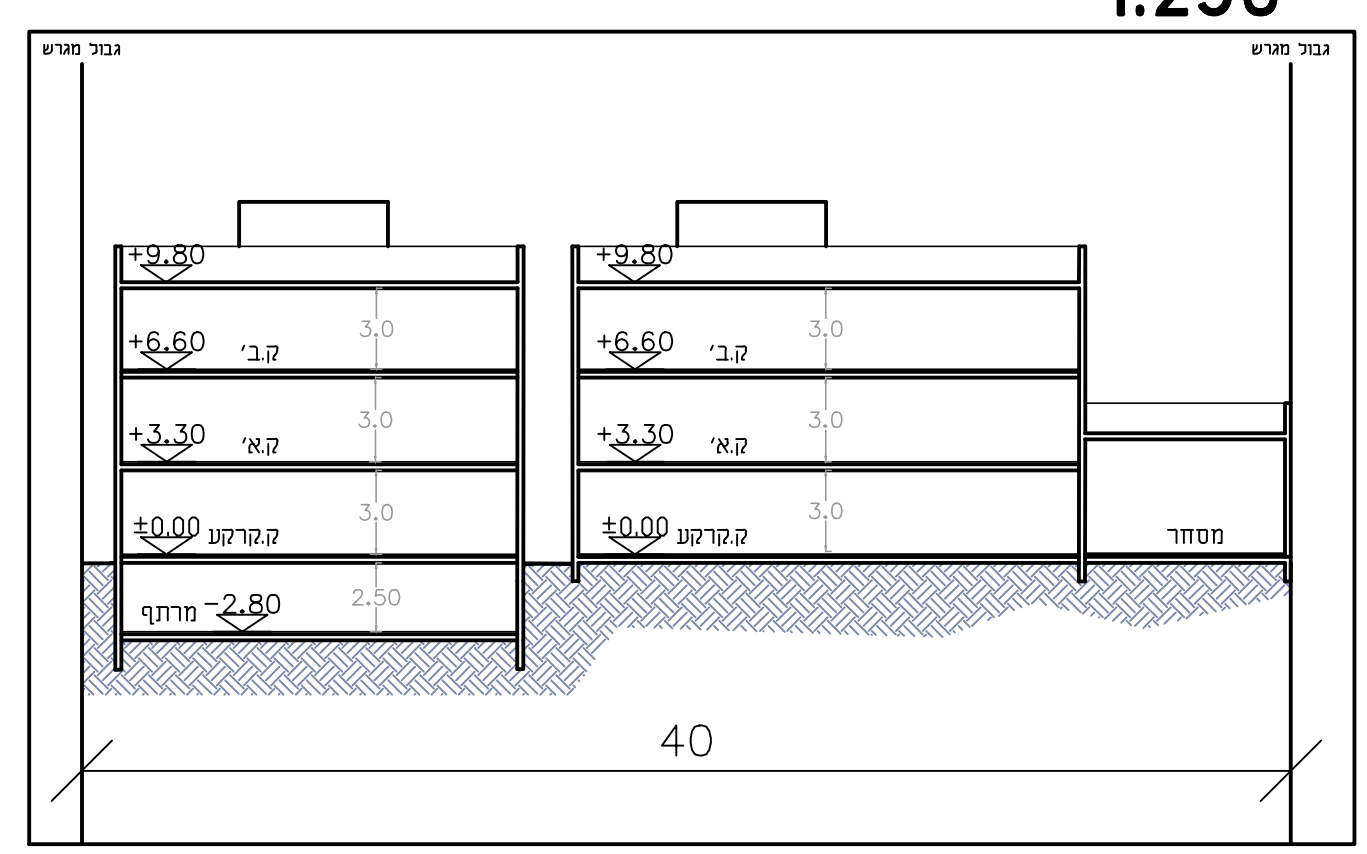
חתך טיפוסי B-B 1:250
