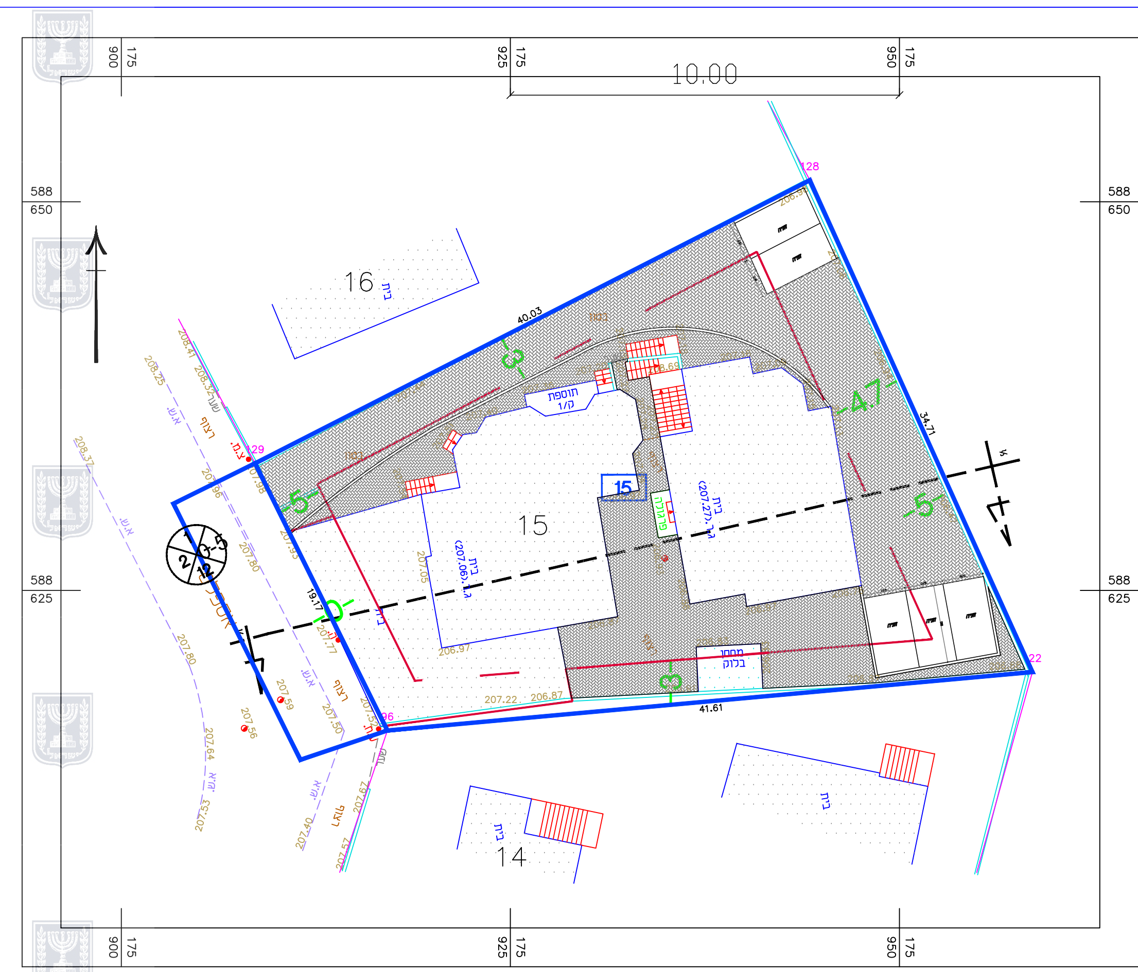
תכנית בנוי סכימטית למגרש 15 בשכונה 22 רהט 1:250
