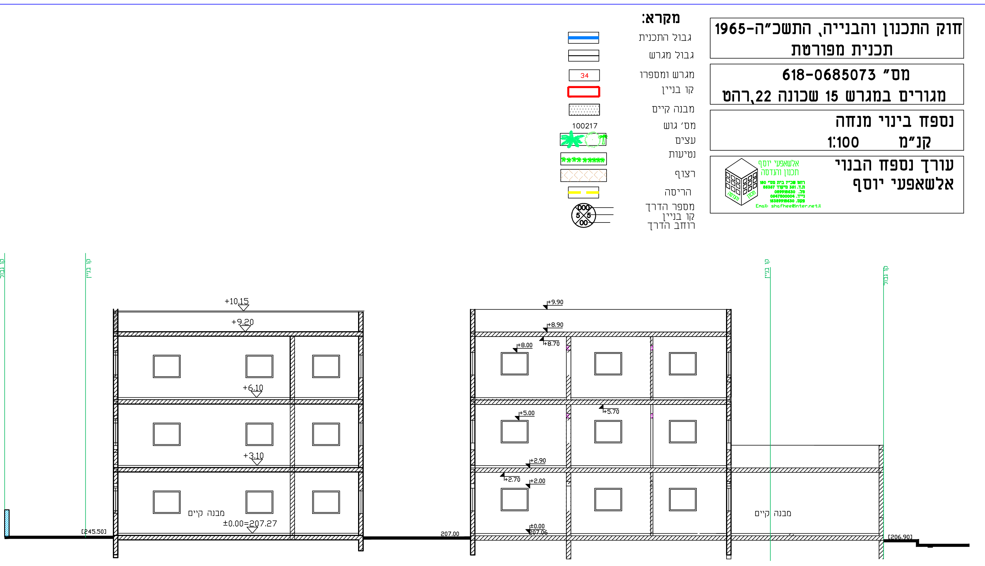
חתך ר-ר 1:100
