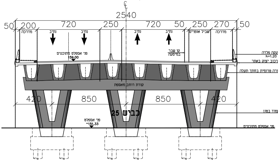
חתך 2-2 לרוחב הגשר מבט על נציבי ביניים - חתך 215
