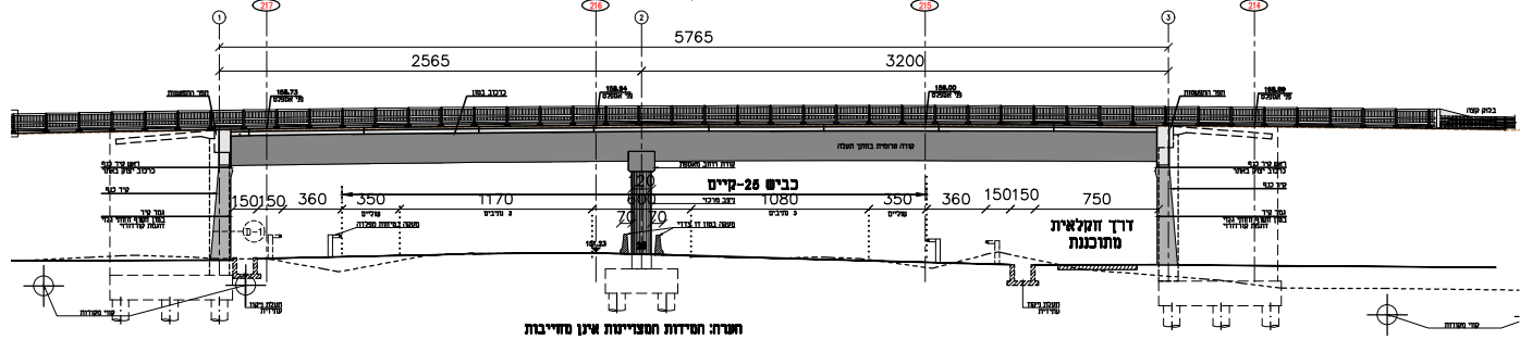
חתך 3-3 לאורך גשר - חתך 2541
