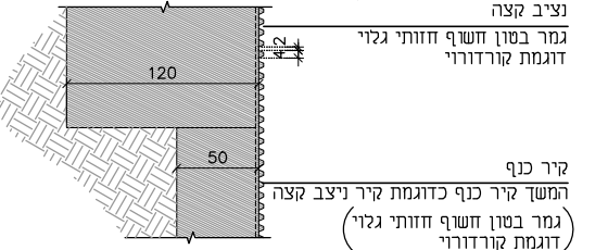
מפגש נציב קצה קיר כנף
