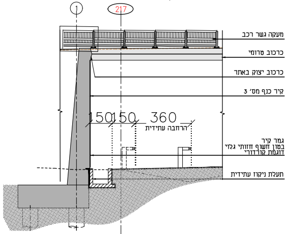
חתך 4-4 קיר כנף מס' 3 - חתך 2542
