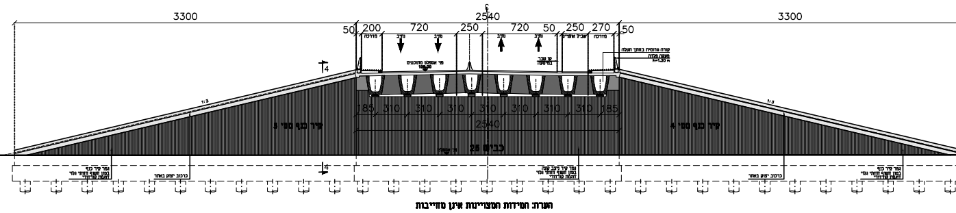
חתך 2-2 לרוחב הגשר מבט על נציבי ביניים - חתך 215
