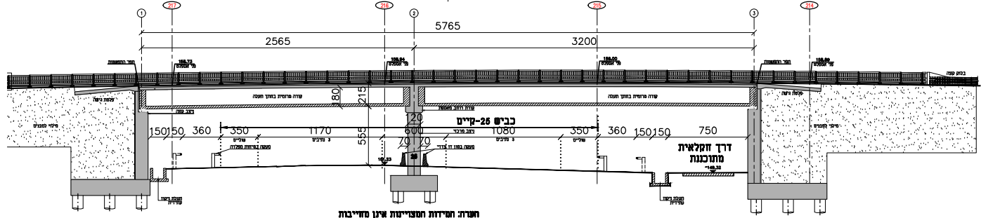
חתך מבט 1-1 נציב קצה ציר 1 - חתך 217
