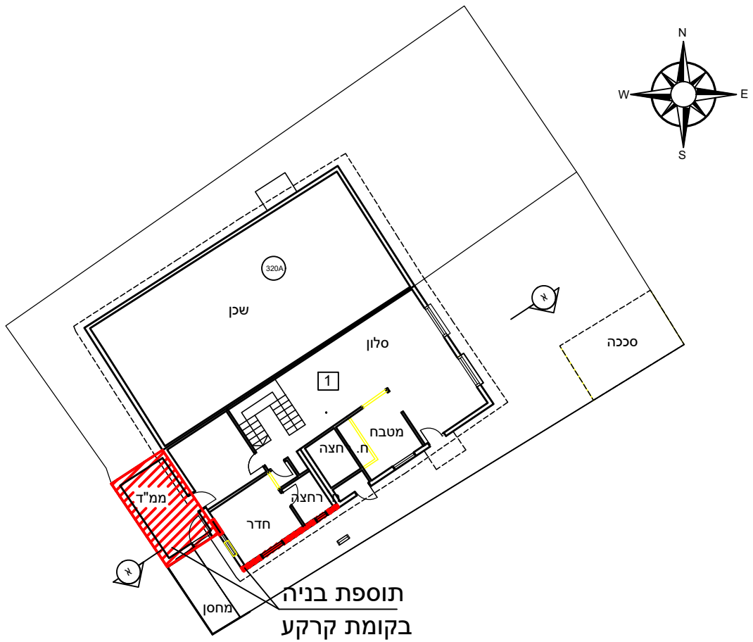
תכנית קומת קרקע קנ"מ 1:250
