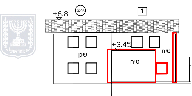
חזית מערבית קנ"מ 1:250
