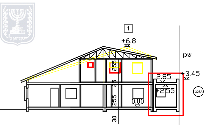
א-א חתך 1:250 קנ"ח
