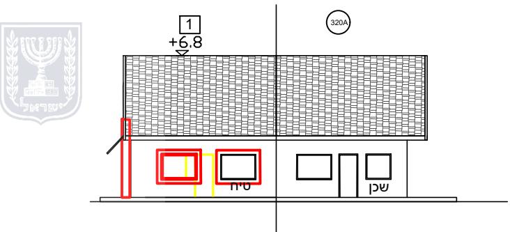
חזית מזרחית קנ"מ 1:250
