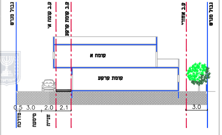
חתך א - א קני"מ 1:100
