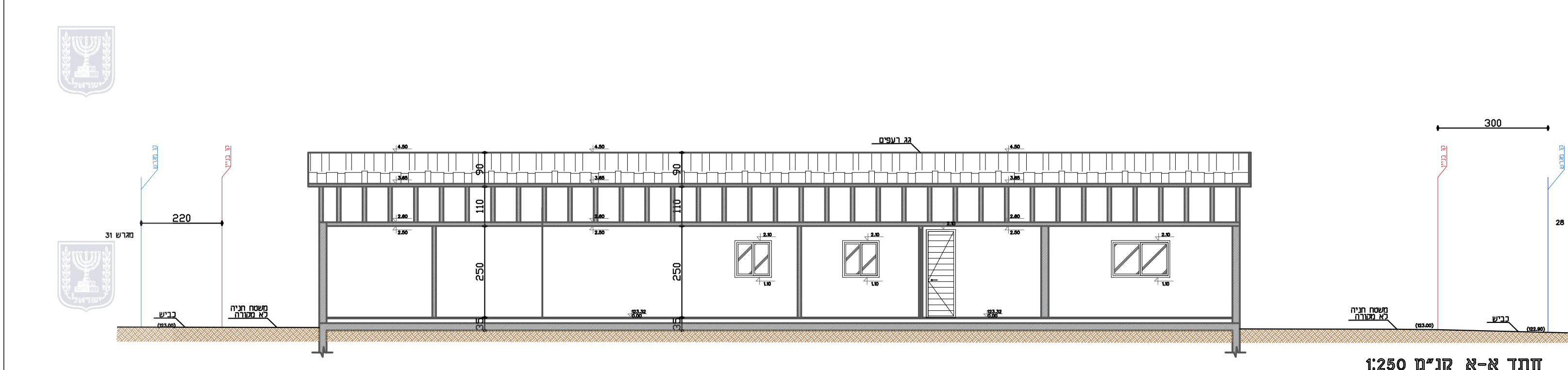
חותך א-א קנ"מ 1:250
