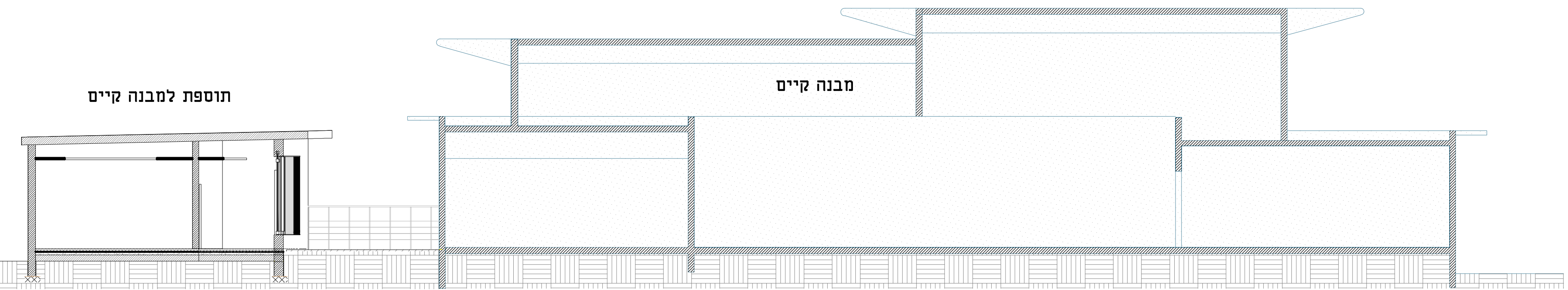
חיתוך א-א
