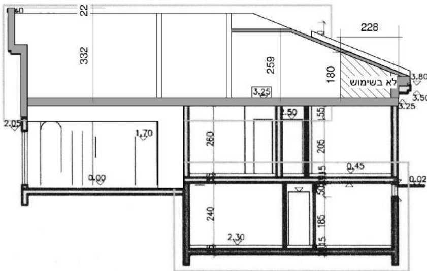
חתך ב-ב קני"מ 1:150
