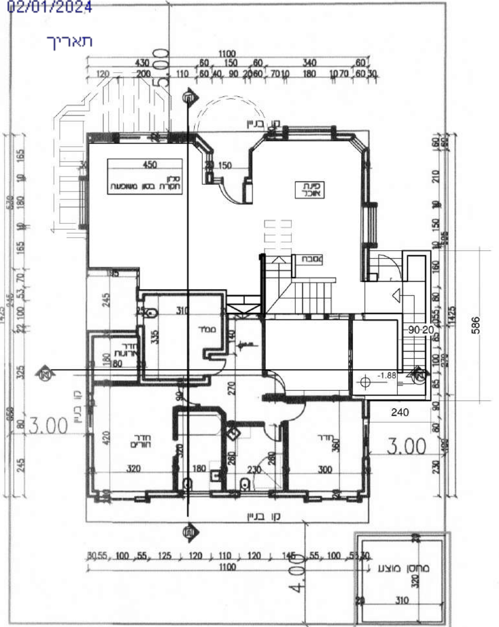
תכנית קומת קרקע קני"מ-150 : 1
