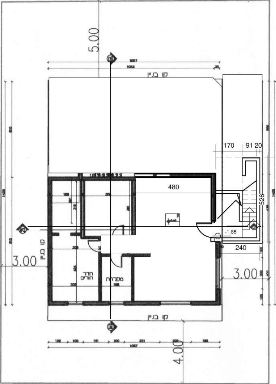
תכנית קומת מרתף קני"מ-150 : 1
