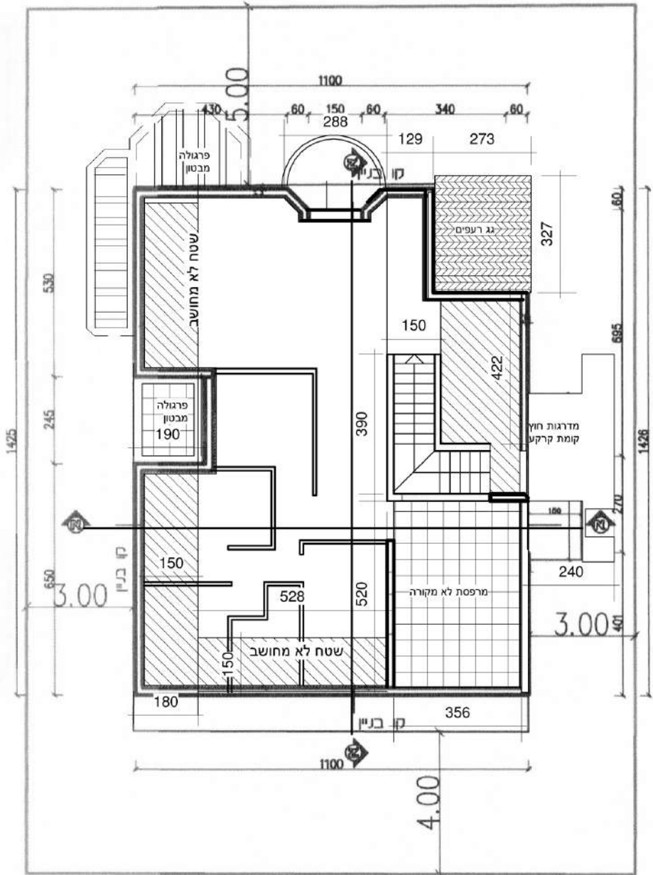
תכנית קומת 3 קני"מ-150 : 1
