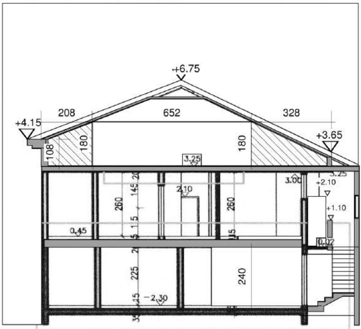
חתך א-א קני"מ 1:150
