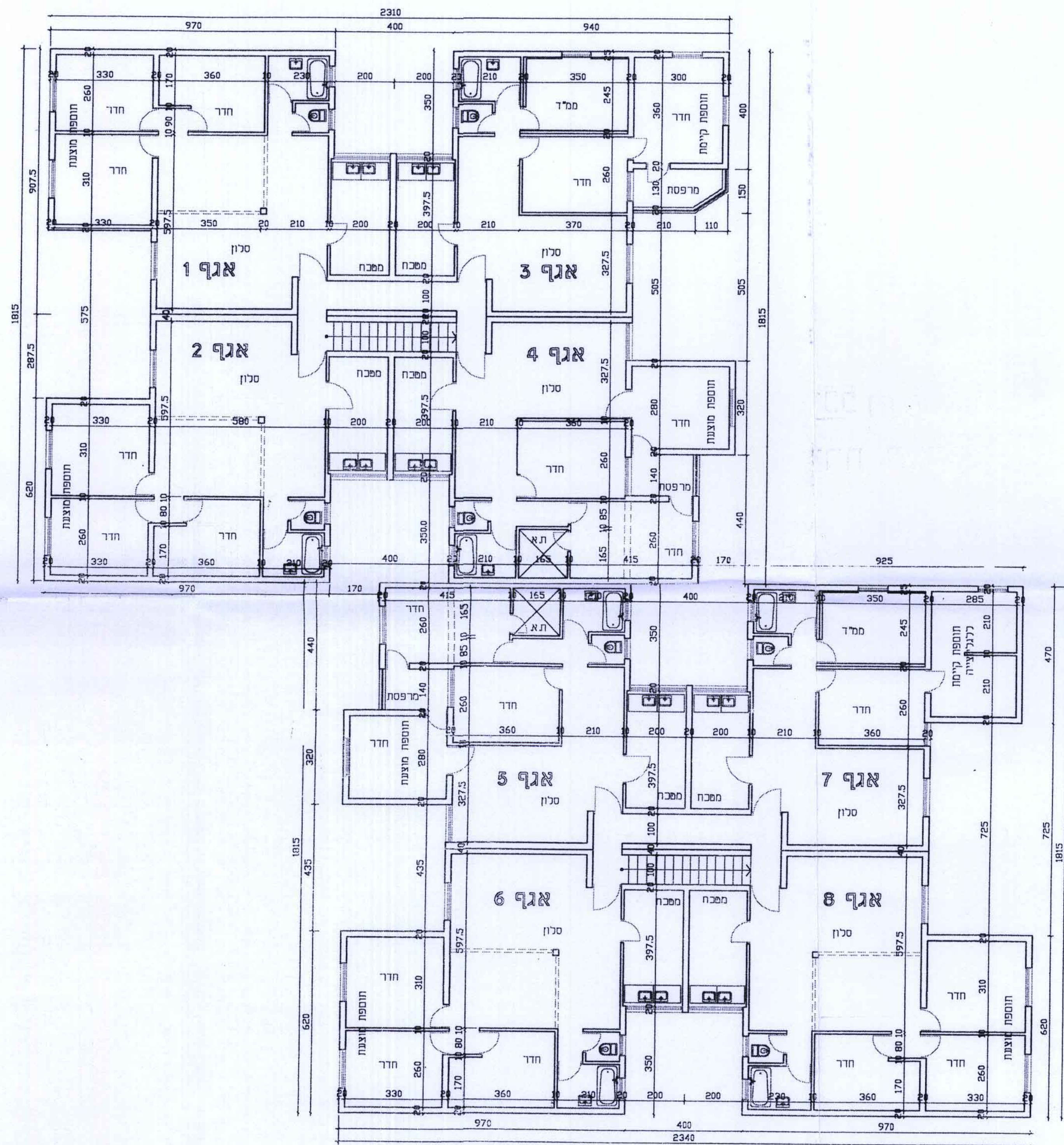
תכנית קומה טיפוסית קנ"מ 1:100
