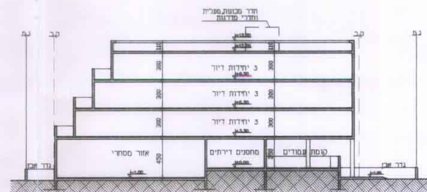
חתך עיקרני א - א ק"מ 1:250
