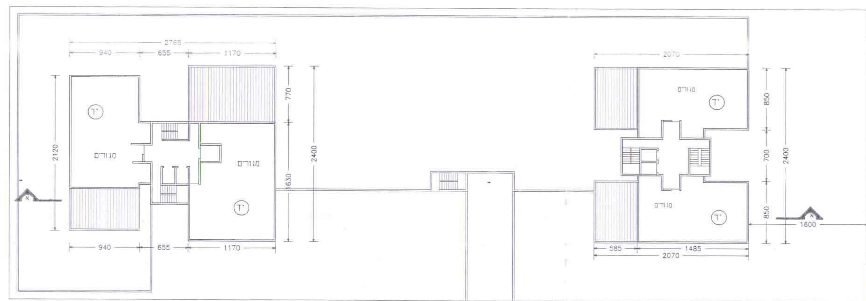
תוכנית קומה י"ד קנ"מ 1:250
